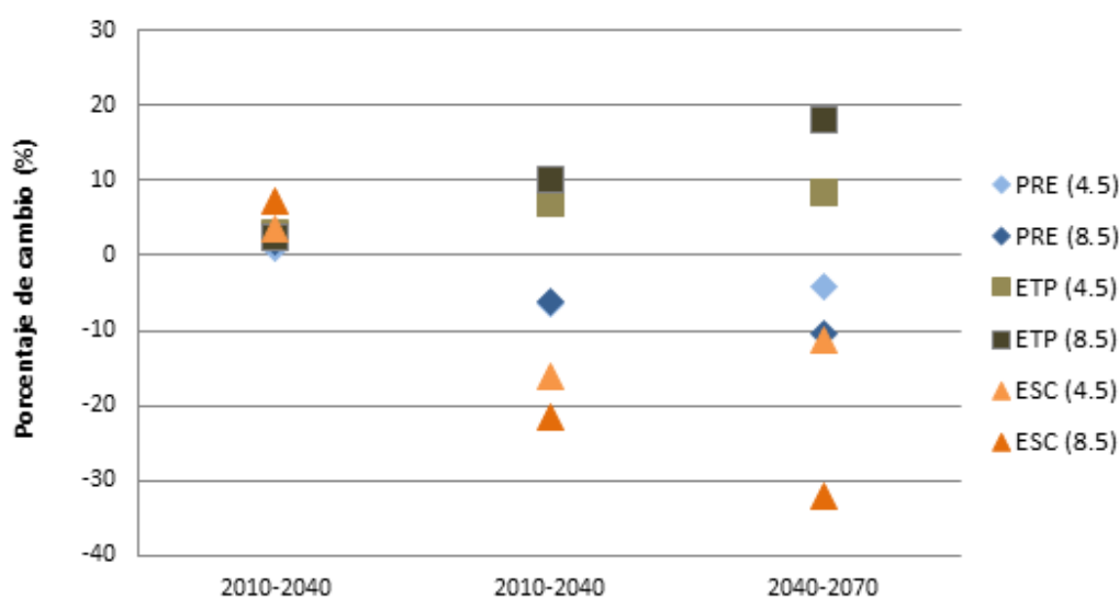
Figura 2: Representación gráfica de porcentaje de cambio con respecto al periodo control y escenarios RCP aplicados a la RNF del Arroyo de Riocamba para las variables de precipitación (PRE), evapotranspiración potencial (ETP) y escorrentía (ESC) con respecto al periodo de control. Fuente: Elaboración propia a partir de la aplicación informática CAMREC versión 1.0 (julio de 2017) desarrollada por el CEDEX.
