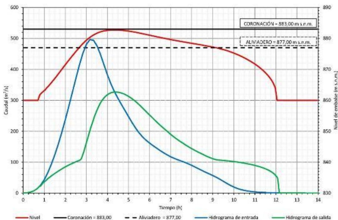
Figura 91. Laminación de la avenida extrema ( T = 5.000 años) en la presa propuesta
