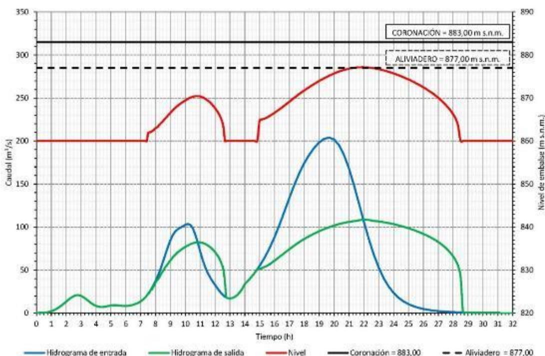
Figura 92. Laminación del evento ocurrido el día 29 de octubre de 2024 en la presa propuesta
