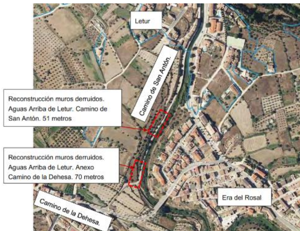
Figura 13. Zonas de desbordamiento del cauce a la carretera San Antón que han requerido la reconstrucción de los muros colapsados. Fuente: Obra de emergencia de los trabajos de retirada de arrastres y reparación del encauzamiento del arroyo Letur. CHS
