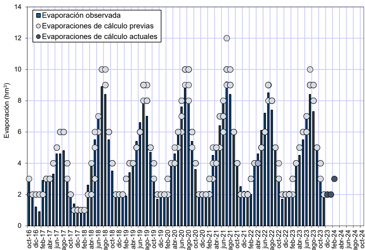
Figura 26. Evaporaciones en Entrepeñas y Buendía observadas y de cálculo.
