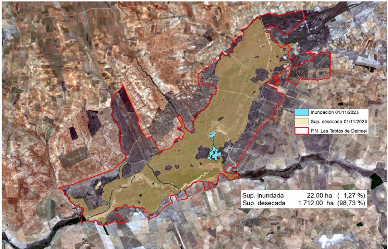
Figura 14. Imagen de la zona inundada del Parque Nacional de las Tablas de Daimiel (1 de noviembre de 2023).
