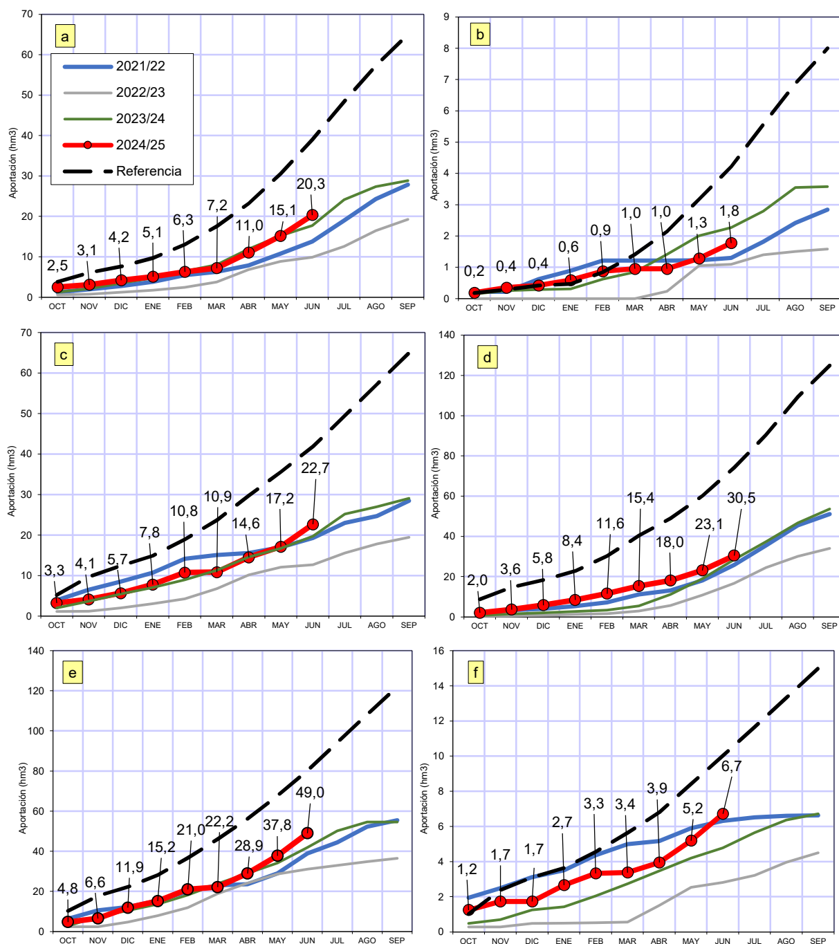
Figura 19. Consumos de las aguas trasvasadas destinadas a riego desde 2020/21 reales y de referencia acumulados mensualmente: a) Vega alta y media del Segura; b) Regadíos de Mula y su comarca; c) Lorca y Valle del Guadalentín; d) Riegos de Levante, margen izquierda y derecha, vegas bajas del Segura y saladares de Alicante; e) Campos de Cartagena; f) Valle del Almanzora, en Almería.
