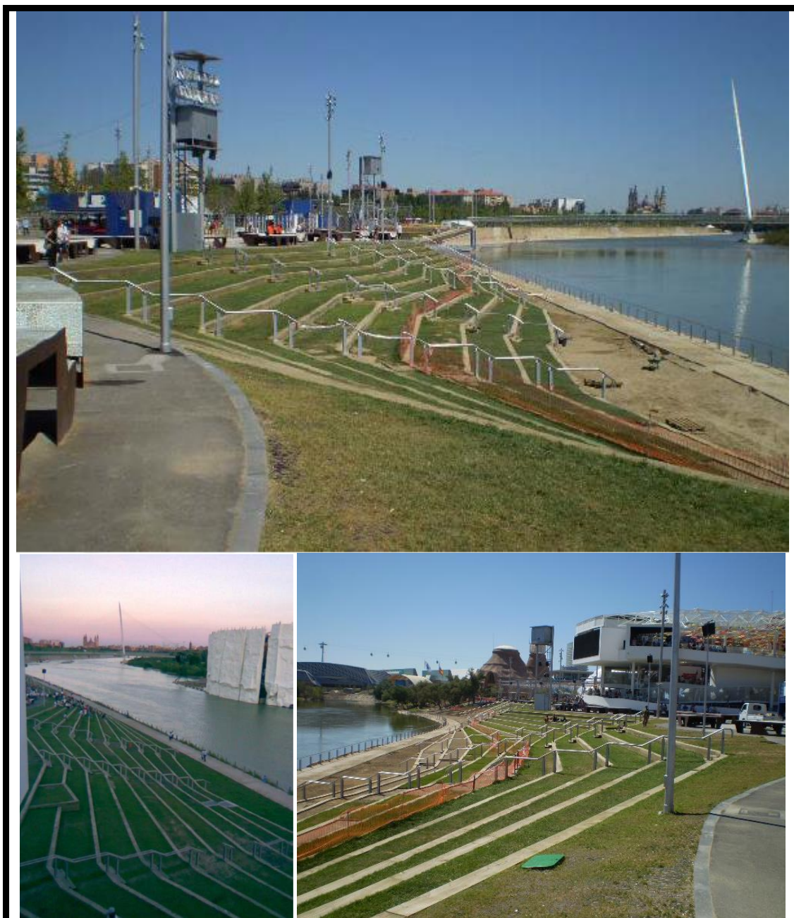
Celdas drenantes de 52 mm (pavimento vegetado) en Graderíos. Expo-Zaragoza. Años 2007-2008. Cortesía de «SUDS S.L - Atlantis».
