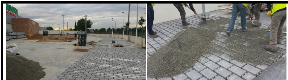
Ecoparking. Palma de Mallorca (España). Drenaje horizontal y acabado final con adoquines. Cortesía de «SUDS S.L - Atlantis».
