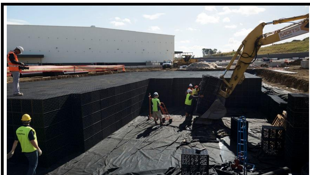
El agua previamente filtrada en los SUDS puede ser almacenada en depósitos. Depósito modular permeable constituido con cajas drenantes envueltas en geotextil. Cortesía de «SUDS S.L - Atlantis».
