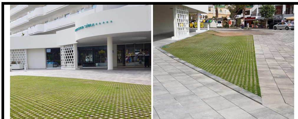
Pavimentos permeables (o drenantes). Pieza que crea una superficie de césped a la vez que soporta las cargas de vehículos. Cortesía de Breinco.
