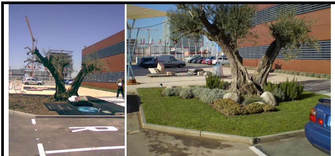
Celdas drenantes de 52 mm en superficie alcorques. Expo-Zaragoza. Años 2007-2008. Cortesía de «SUDS S.L - Atlantis».
