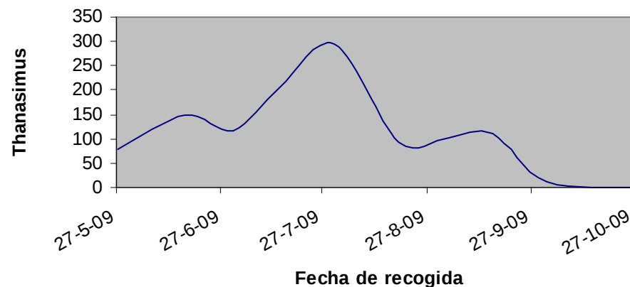
Curva de vuelo de Thanasimus en la Cerdanya. Año 2009
