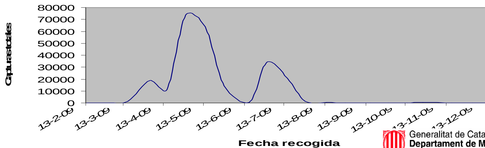
Curva de vuelo de Ips acuminatus en el aserradero Can Boix, año 2009
