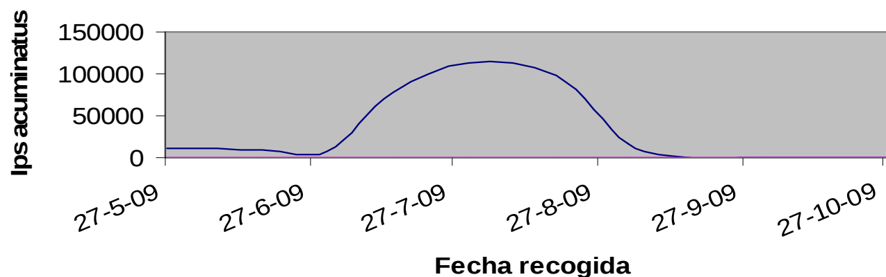
Curva de vuelo de Ips acuminatus en la Cerdanya. Año 2009
