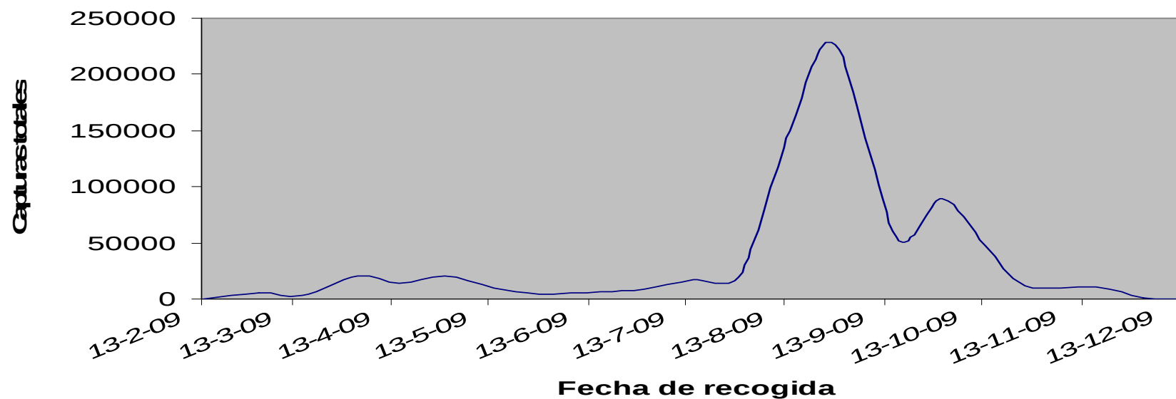
Curva de vuelo de Ips acuminatus en el aserradero Can Boix, año 2009
