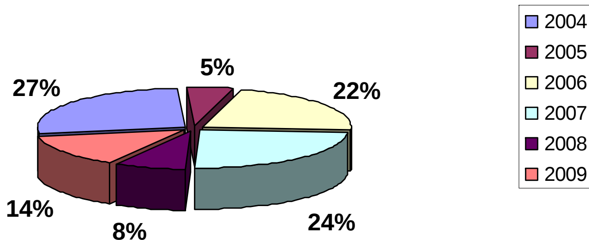
Capturas anuales de Ips Sexdentatus en Can Olivé
