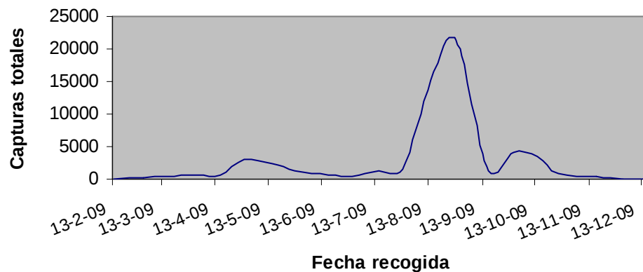
Curva de vuelo de Ips sexdentatus en Puig Reig, año 2009
