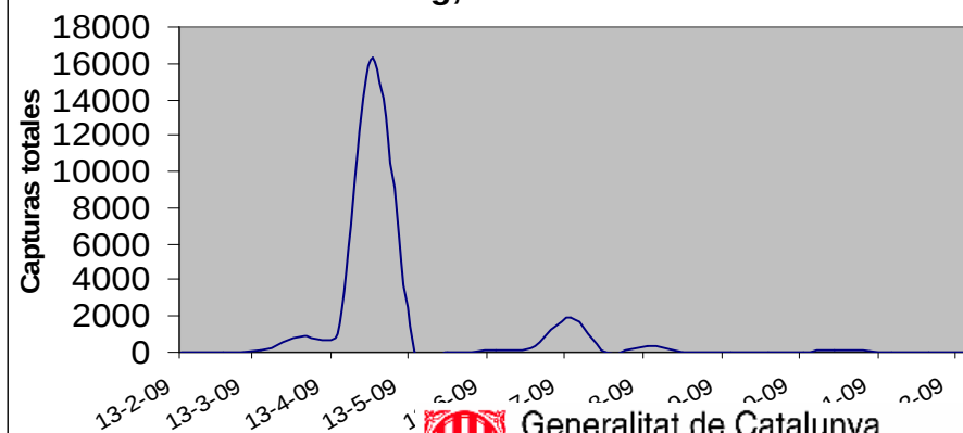
Curva de vuelo de Ips acuminatus en Puig Reig, año 2009
