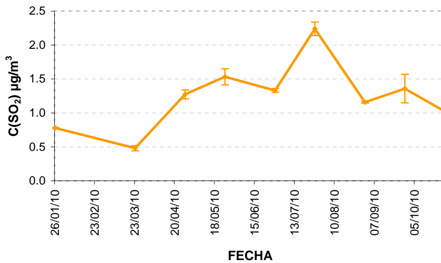
Figura 36: Concentraciones de Dióxido de Azufre (SO 2 µg/m 3 ) durante el año 2010 en la parcela de Andujar.
