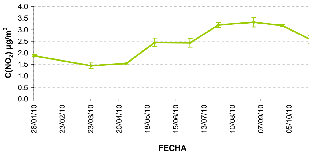
Figura 35: Concentraciones de Dióxido de Nitrógeno (NO 2 µg/m 3 ) en el año 2010 en la parcela de Andujar.
