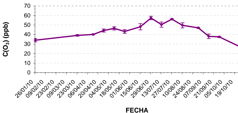
Figura 34: Concentraciones de ozono (ppb) en el año 2010 en la parcela de Andujar.
