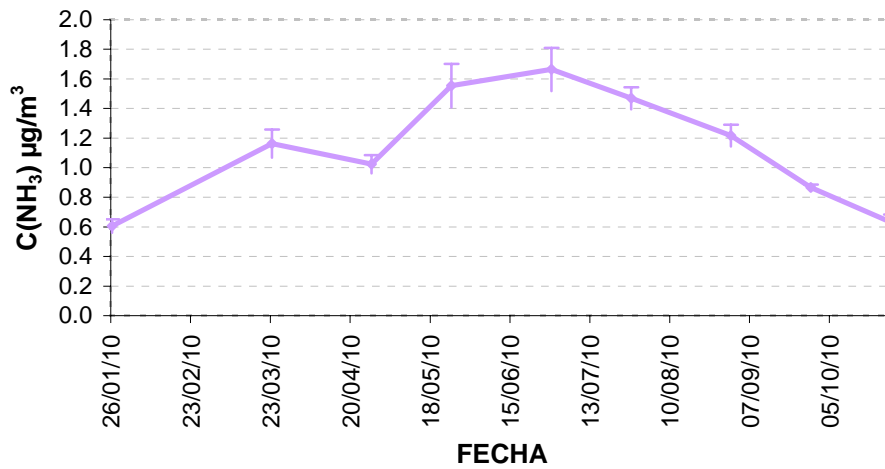
Figura 37: Concentraciones de Amoniac (NH 3 µg/m 3 ) entre durante el año 2010 en la parcela de Andujar.
