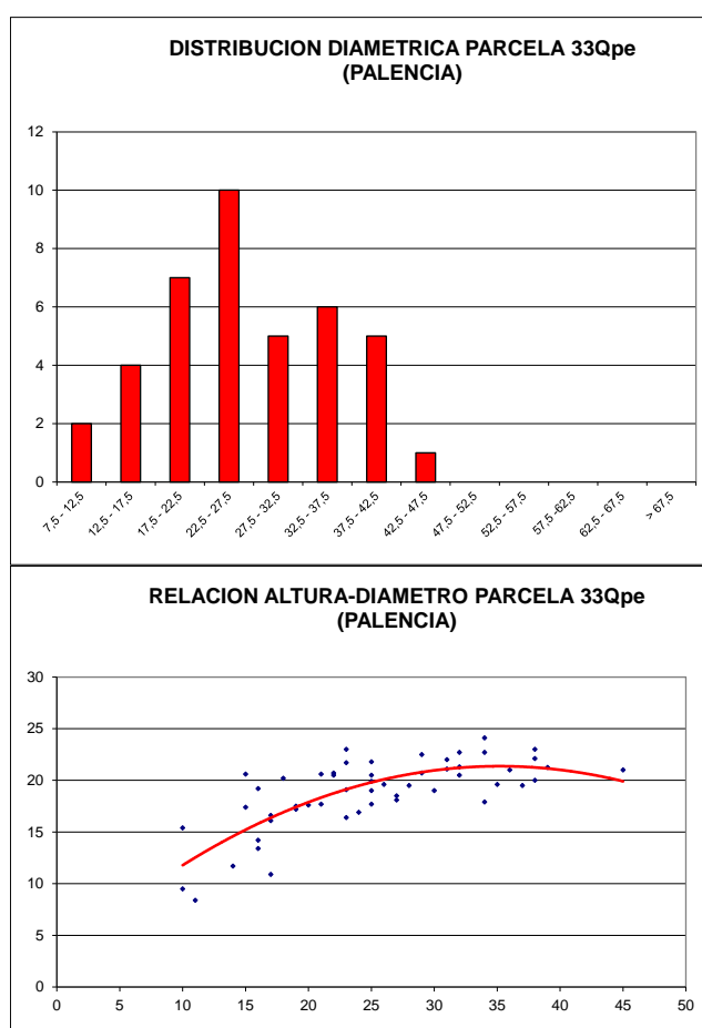
FIG 3: Distribución diamétrica de la parcela; distribución de alturas y comparación con las alturas media y dominante; relación de alturas-diámetros; frecuencias, alturas, esbelteces y existencias por clase diamétrica.
