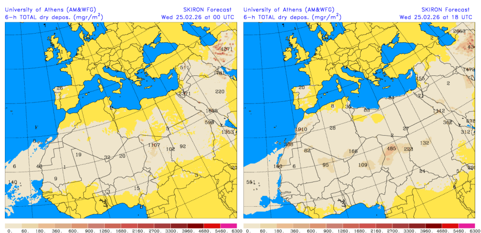
Depósito seco de polvo ( \text{mg}/\text{m}^2 ) predicho por el modelo SKIRON para el día 25 de febrero de 2026 a las 00 y 18 UTC © Universidad de Atenas.
