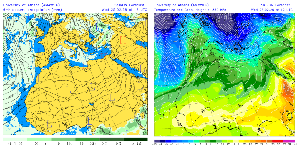
Precipitación acumulada (mm) y presión a nivel del mar (hPa) (izquierda) y campo de temperaturas (°C) y de altura geopotencial a 850 hPa (derecha) previsto por el modelo SKIRON para el día 25 de febrero de 2026 a las 12 UTC © Universidad de Atenas.
