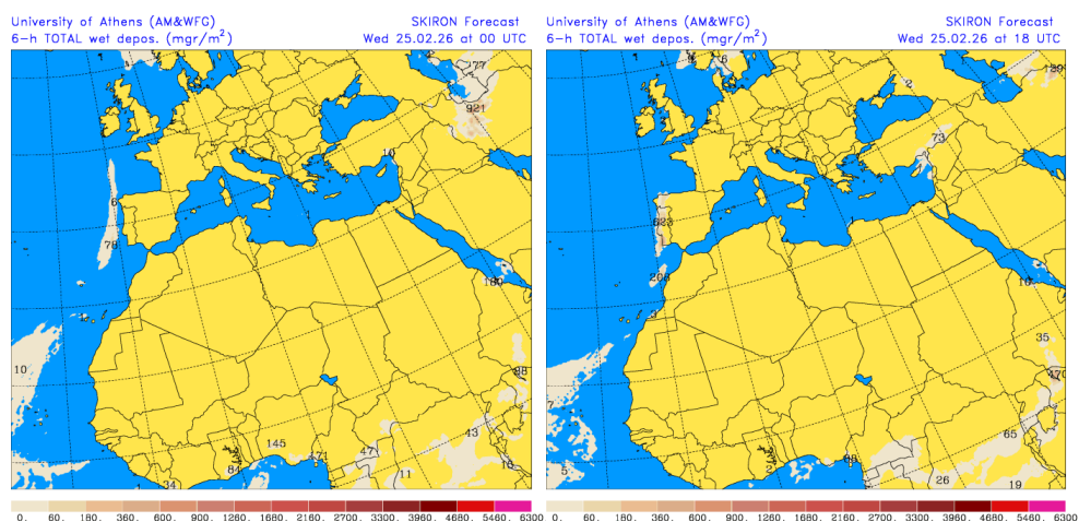
Depósito húmedo de polvo ( \text{mg}/\text{m}^2 ) predicho por el modelo SKIRON para el día 25 de febrero de 2026 a las 00 y 18 UTC © Universidad de Atenas.
