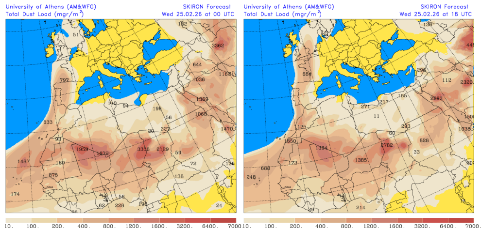
Carga total de polvo (mg/m 2 ) predicha por el modelo SKIRON para el día 25 de febrero de 2026 a las 00 y 18 UTC © Universidad de Atenas.
