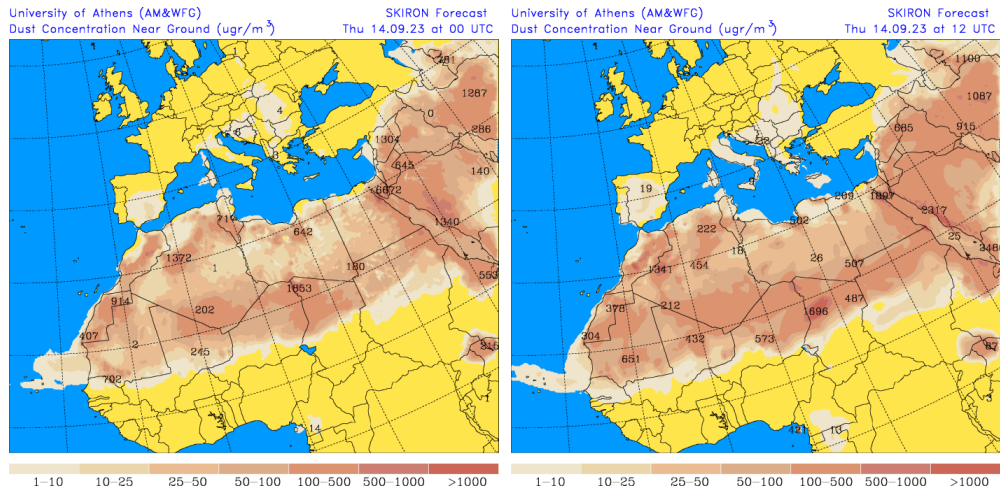
Concentración de polvo ( \mu\text{g}/\text{m}^3 ) predicha por el modelo SKIRON para el día 14 de septiembre de 2023 a las 00 y 12 UTC © Universidad de Atenas.
