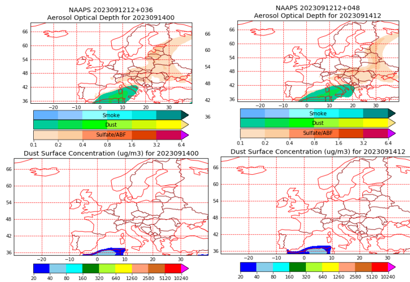
Espesor óptico de aerosoles a 550 nm (arriba) y concentración de polvo a nivel de superficie (abajo) previstos por el modelo NAAPS para el día 14 de septiembre de 2023 a las 00 h UTC y a las 12 h UTC. ©Naval Research Laboratory (NRL), Monterey, CA.
