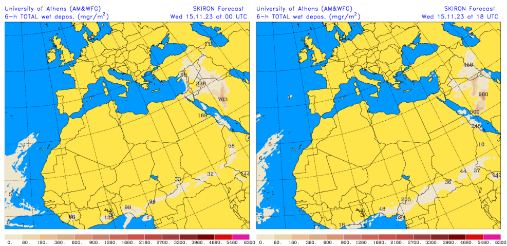
Depósito húmedo de polvo ( \text{mg}/\text{m}^2 ) predicho por el modelo SKIRON para el día 15 de noviembre de 2023 a las 00 y 18 UTC © Universidad de Atenas.
