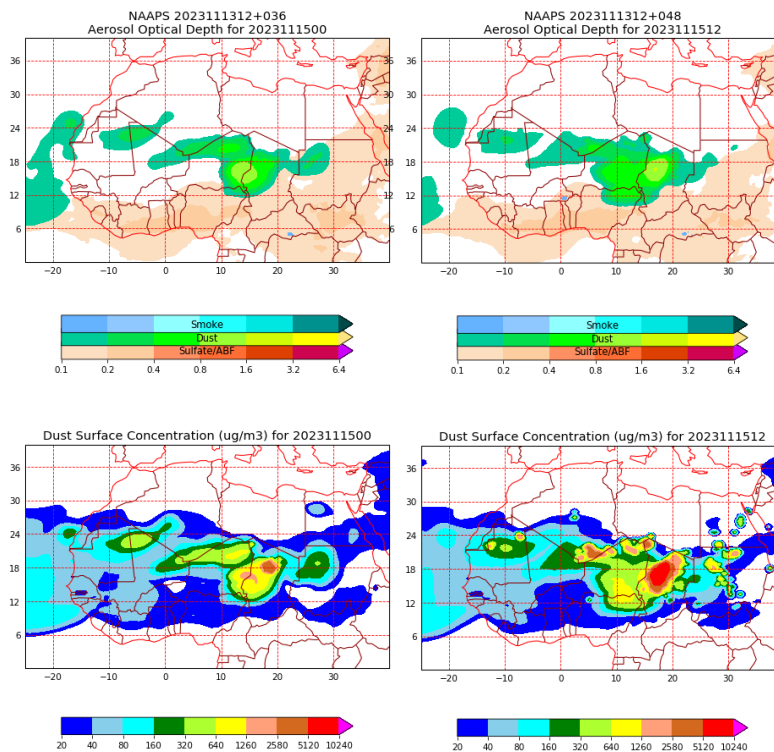
Espesor óptico de aerosoles a 550 nm (arriba) y concentración de polvo a nivel de superficie (abajo) previstos por el modelo NAAPs para el día 15 de noviembre de 2023 a las 00 h UTC y a las 12 h UTC. ©Naval Research Laboratory (NRL), Monterey, CA.
