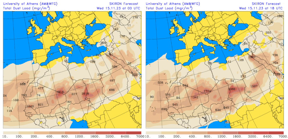
Carga total de polvo (mg/m 2 ) predicha por el modelo SKIRON para el día 15 de noviembre de 2023 a las 00 y 18 UTC © Universidad de Atenas.
