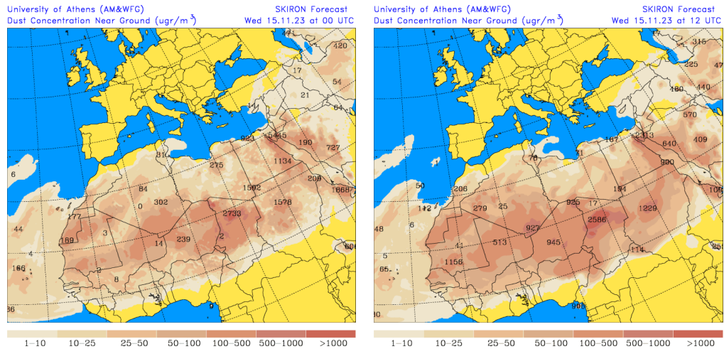
Concentración de polvo ( \mu\text{g}/\text{m}^3 ) predicha por el modelo SKIRON para el día 15 de noviembre de 2023 a las 00 y 12 UTC © Universidad de Atenas.
