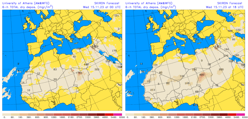
Depósito seco de polvo ( \text{mg}/\text{m}^2 ) predicho por el modelo SKIRON para el día 15 de noviembre de 2023 a las 00 y 18 UTC © Universidad de Atenas.
