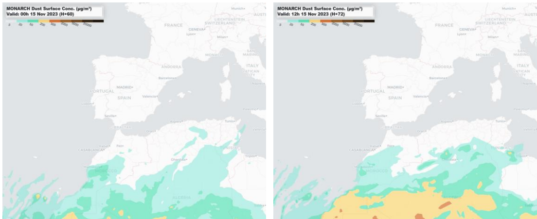
Concentración de polvo ( \mu\text{g}/\text{m}^3 ) predicha por el modelo MONARCH para el día 15 de noviembre de 2023 a las 00h y 12h UTC. © Barcelona Dust Regional Center.
