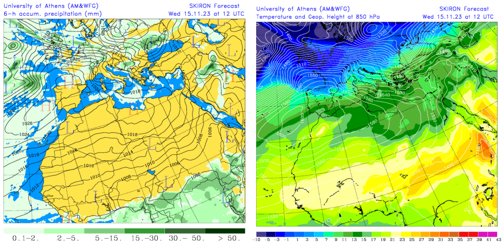
Precipitación acumulada (mm) y presión a nivel del mar (hPa) (izquierda) y campo de temperaturas (°C) y de altura geopotencial a 850 hPa (derecha) previsto por el modelo SKIRON para el día 15 de noviembre de 2023 a las 12 UTC © Universidad de Atenas.
