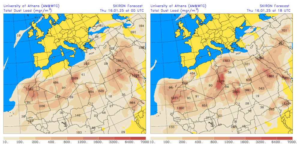
Carga total de polvo ( \text{mg}/\text{m}^2 ) predicha por el modelo SKIRON para el día 16 de enero de 2025 a las 00 y 18 UTC © Universidad de Atenas.
