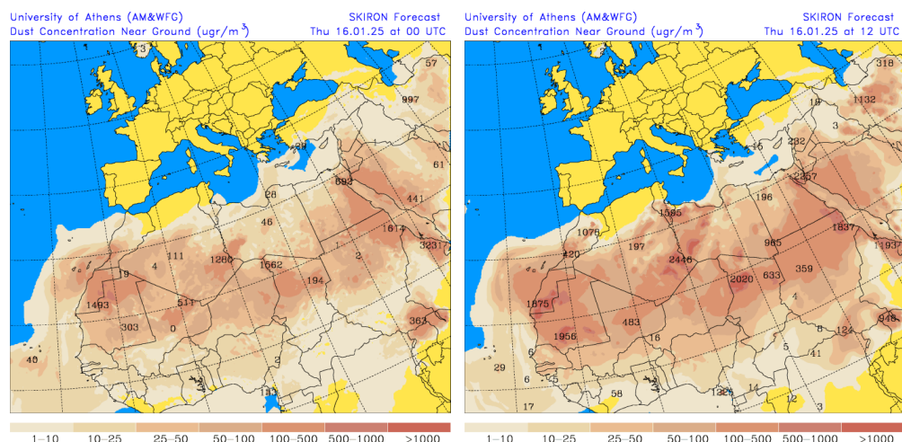
Concentración de polvo ( \mu\text{g}/\text{m}^3 ) predicha por el modelo SKIRON el día 16 de enero de 2025 a las 00 y 12 UTC © Universidad de Atenas.
