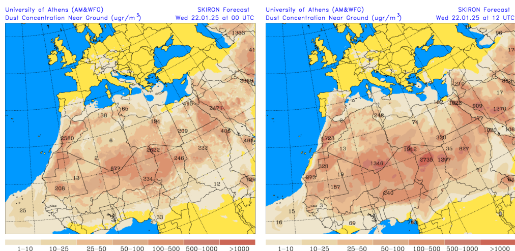
Concentración de polvo ( \mu\text{g}/\text{m}^3 ) predicha por el modelo SKIRON el día 22 de enero de 2025 a las 00 y 12 UTC © Universidad de Atenas.
