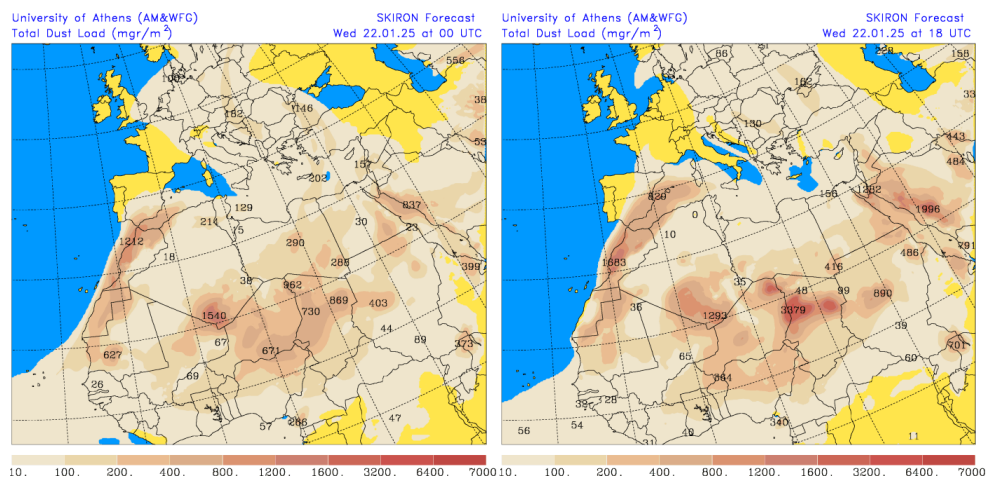
Carga total de polvo ( \text{mg}/\text{m}^2 ) predicha por el modelo SKIRON para el día 22 de enero de 2025 a las 00 y 18 UTC © Universidad de Atenas.
