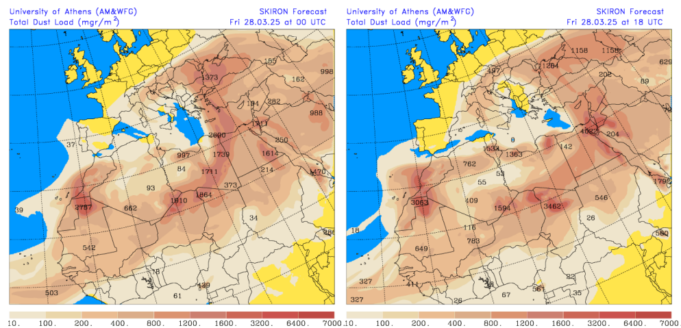
Carga total de polvo ( \text{mg}/\text{m}^2 ) predicha por el modelo SKIRON para el día 28 de marzo de 2025 a las 00 y 18 UTC © Universidad de Atenas.
