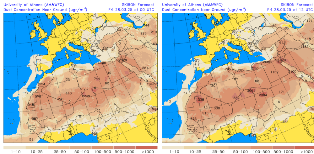
Concentración de polvo ( \mu\text{g}/\text{m}^3 ) predicha por el modelo SKIRON para el día 28 de marzo de 2025 a las 00 y 12 UTC © Universidad de Atenas.
