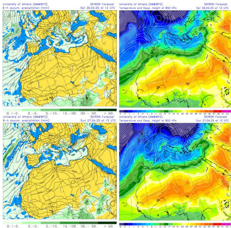
Precipitación acumulada (mm) y presión a nivel del mar (hPa) (izquierda) y campo de temperaturas (°C) y de altura geopotencial a 850 hPa (derecha) previsto por el modelo SKIRON para los días 26 y 27 de abril de 2025 a las 12 UTC © Universidad de Atenas.
