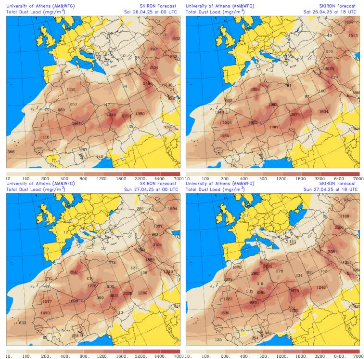
Carga total de polvo (mg/m 2 ) predicha por el modelo SKIRON para los días 26 y 27 de abril de 2025 a las 00 y 18 UTC © Universidad de Atenas.
