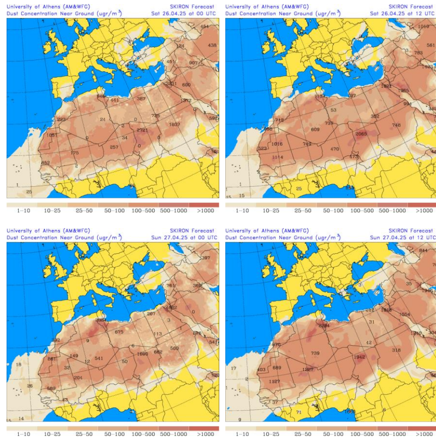
Concentración de polvo ( \mu\text{g}/\text{m}^3 ) predicha por el modelo SKIRON para los días 26 y 27 de abril de 2025 a las 00 y 12 UTC © Universidad de Atenas.
