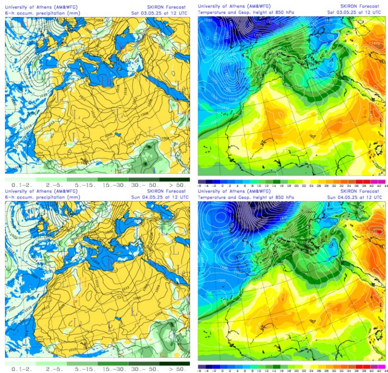
Precipitación acumulada (mm) y presión a nivel del mar (hPa) (izquierda) y campo de temperaturas (°C) y de altura geopotencial a 850 hPa (derecha) previsto por el modelo SKIRON para los días 3 y 4 de mayo de 2025 a las 12 UTC © Universidad de Atenas.
