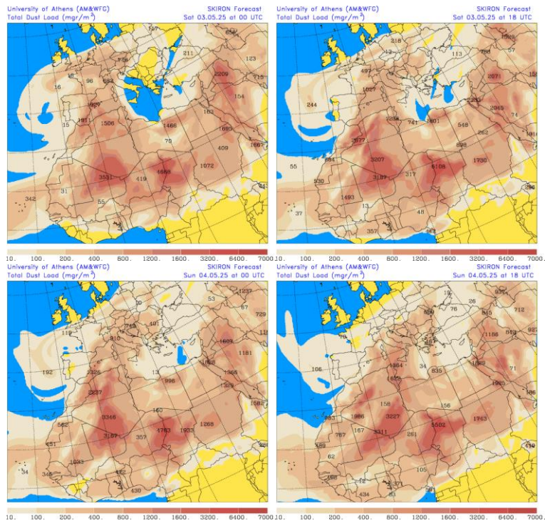
Carga total de polvo (mg/m 2 ) predicha por el modelo SKIRON para los días 3 y 4 de mayo de 2025 a las 00 y 18 UTC © Universidad de Atenas.
