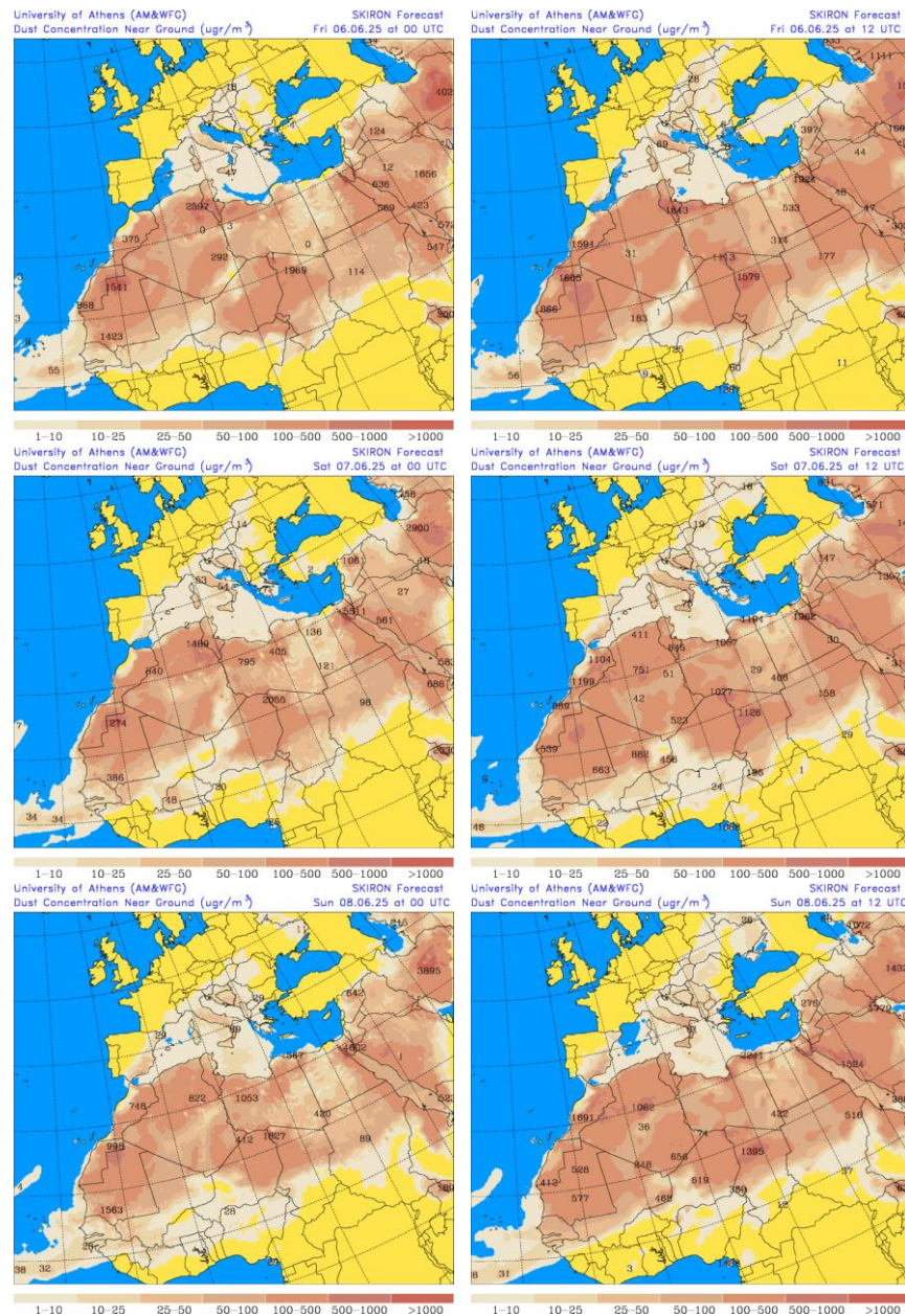
Concentración de polvo ( \mu\text{g}/\text{m}^3 ) predicha por el modelo SKIRON para los días 6, 7 y 8 de junio de 2025 a las 00 y 12 UTC © Universidad de Atenas.
