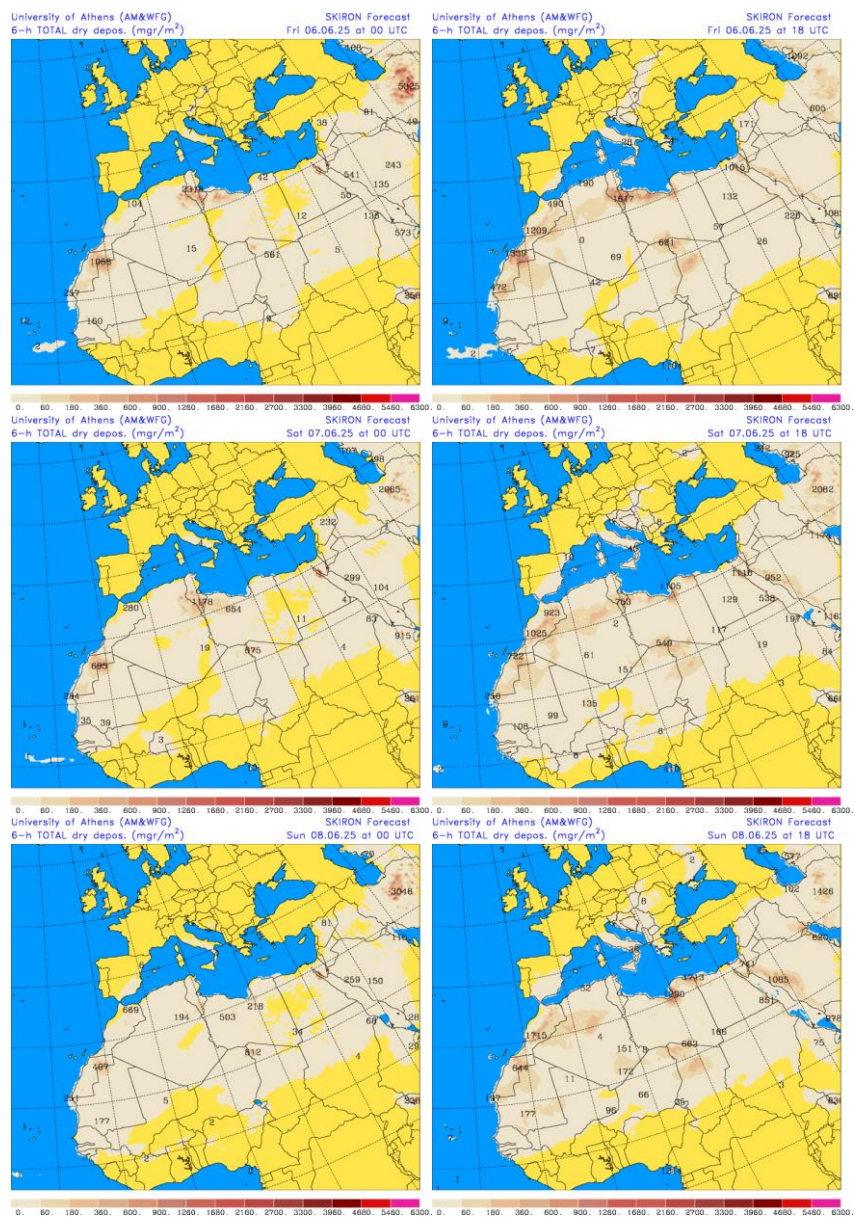
Depósito seco de polvo ( \text{mg}/\text{m}^2 ) predicho por el modelo SKIRON para los días 6, 7 y 8 de junio de 2025 a las 00 y 18 UTC © Universidad de Atenas.
