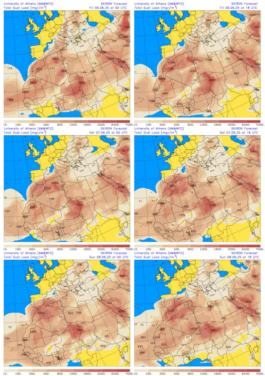
Carga total de polvo (mg/m²) predicha por el modelo SKIRON para los días 6, 7 y 8 de junio de 2025 a las 00 y 18 UTC © Universidad de Atenas.
