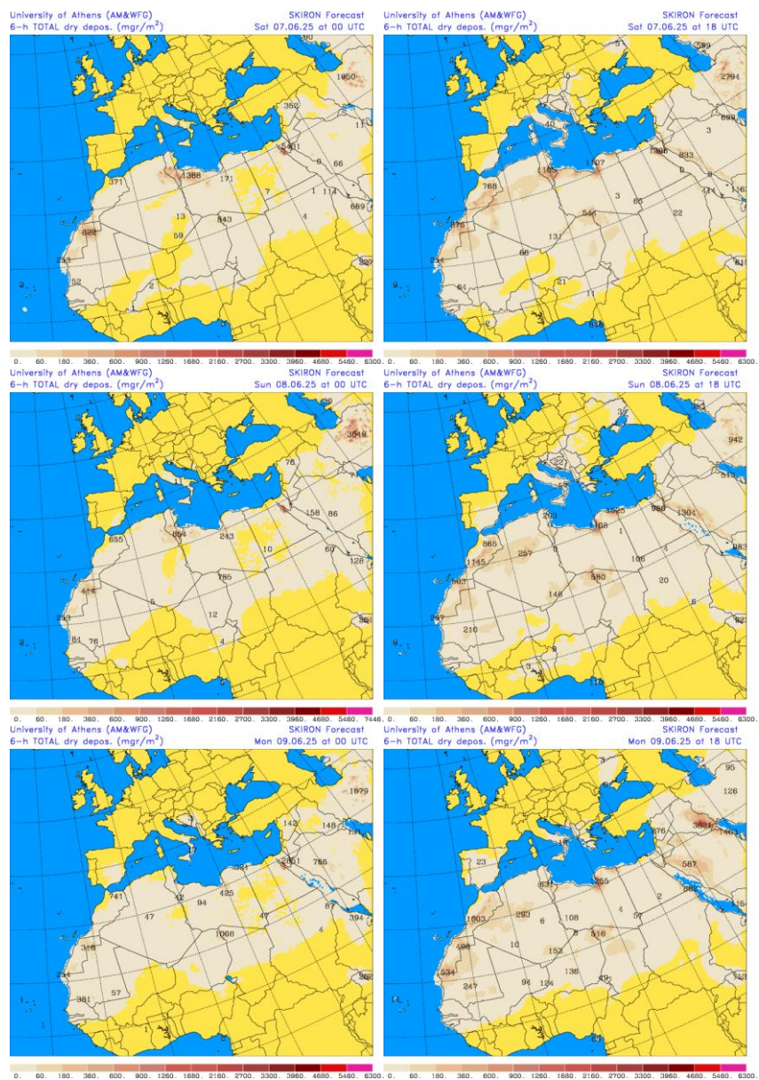
Depósito seco de polvo (mg/m 2 ) predicho por el modelo SKIRON para los días 7, 8 y 9 de junio de 2025 a las 00 y 18 UTC © Universidad de Atenas.
