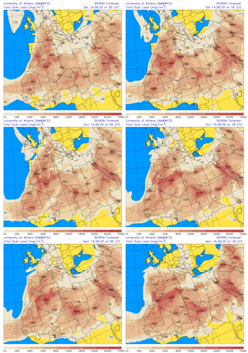
Carga total de polvo (mg/m²) predicha por el modelo SKIRON para los días 14, 15 y 16 de junio de 2025 a las 00 y 18 UTC © Universidad de Atenas.
