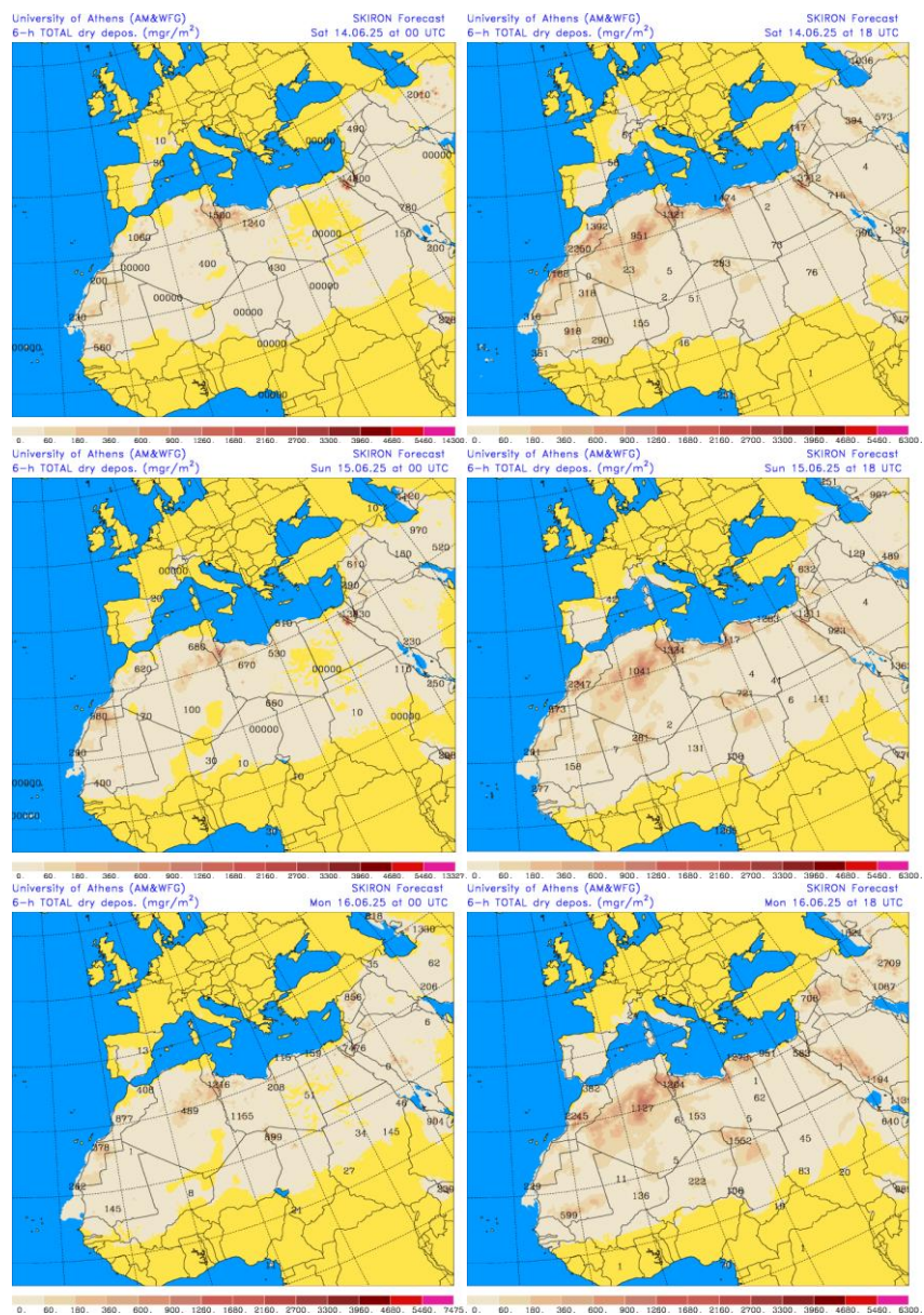
Depósito seco de polvo (mg/m 2 ) predicho por el modelo SKIRON para los días 14, 15 y 16 de junio de 2025 a las 00 y 18 UTC © Universidad de Atenas.
