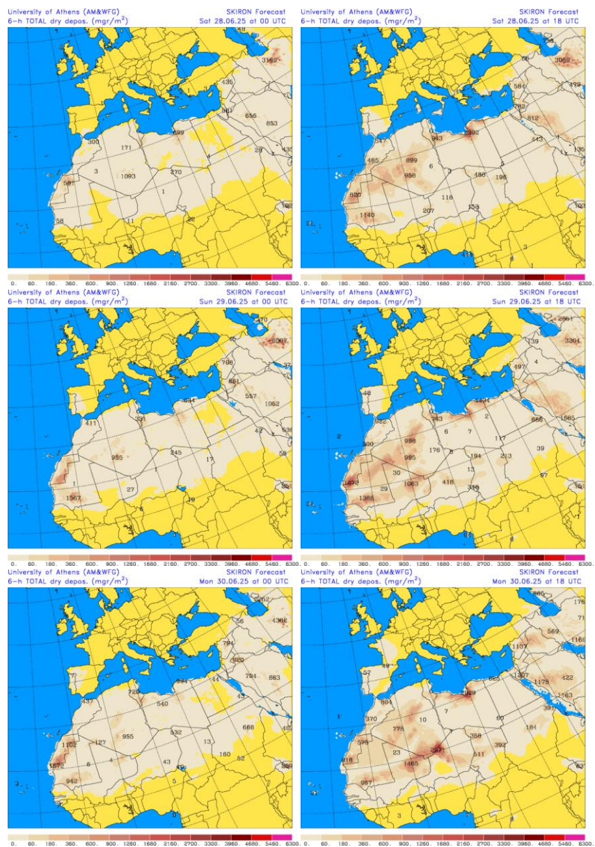
Depósito seco de polvo (mg/m 2 ) predicho por el modelo SKIRON para los días 28, 29 y 30 de junio de 2025 a las 00 y 18 UTC © Universidad de Atenas.
