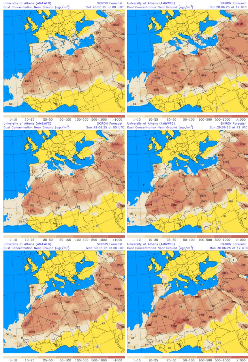
Concentración de polvo ( \mu\text{g}/\text{m}^3 ) predicha por el modelo SKIRON para los días 28, 29 y 30 de junio de 2025 a las 00 y 12 UTC © Universidad de Atenas.
