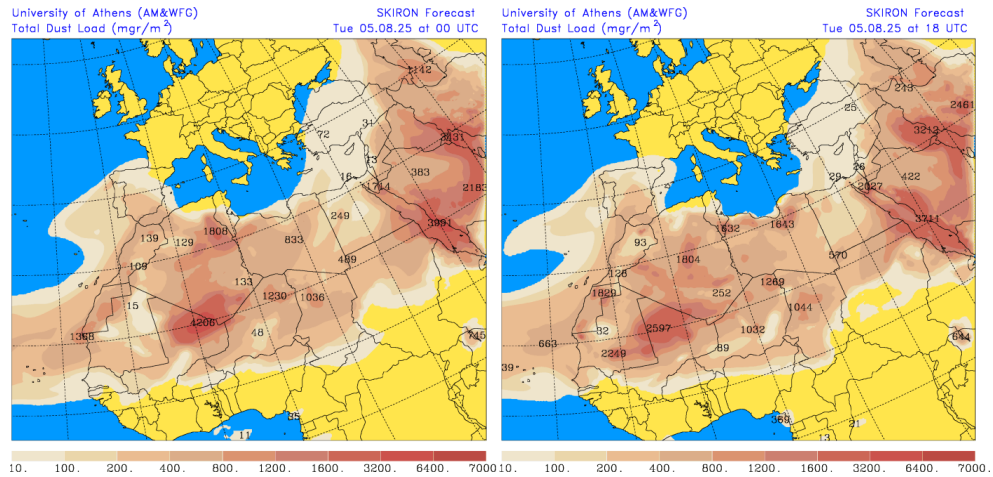
Carga total de polvo (mg/m 2 ) predicha por el modelo SKIRON para el día 5 de agosto de 2025 a las 00 y 18 UTC © Universidad de Atenas.
