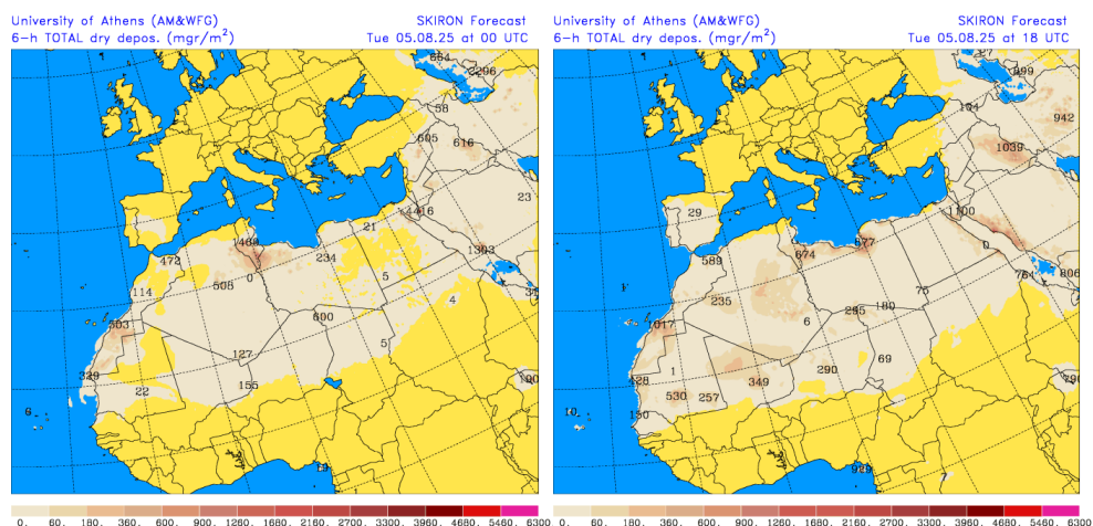
Depósito seco de polvo (mg/m 2 ) predicho por el modelo SKIRON para el día 5 de agosto de 2025 a las 00 y 18 UTC © Universidad de Atenas.
