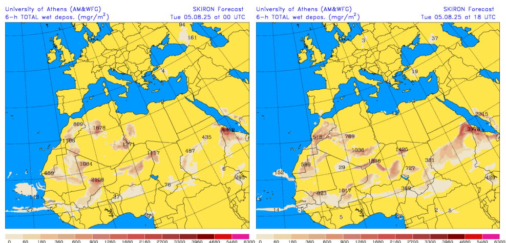
Depósito húmedo de polvo (mg/m 2 ) predicho por el modelo SKIRON para el día 5 de agosto de 2025 a las 00 y 18 UTC © Universidad de Atenas.
