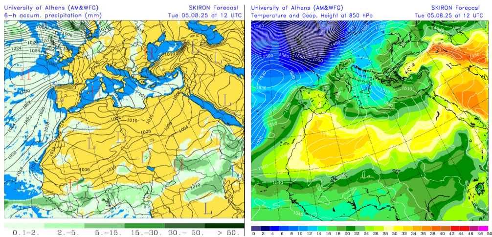
Precipitación acumulada (mm) y presión a nivel del mar (hPa) (izquierda) y campo de temperaturas (°C) y de altura geopotencial a 850 hPa (derecha) previsto por el modelo SKIRON para el día 5 de agosto de 2025 a las 12 UTC © Universidad de Atenas.
