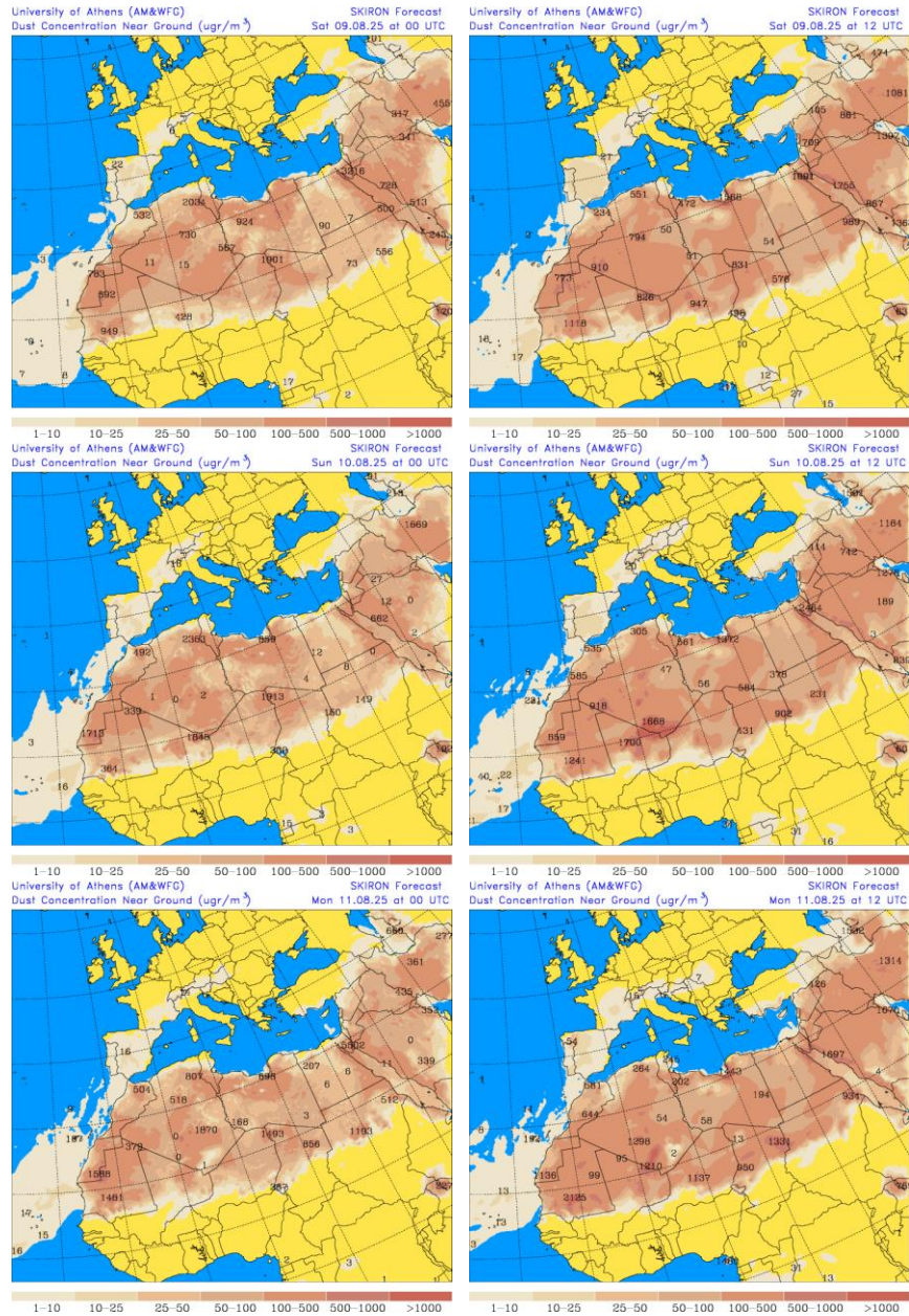
Concentración de polvo ( \mu\text{g}/\text{m}^3 ) predicha por el modelo SKIRON para los días 9, 10 y 11 de agosto de 2025 a las 00 y 12 UTC © Universidad de Atenas.
