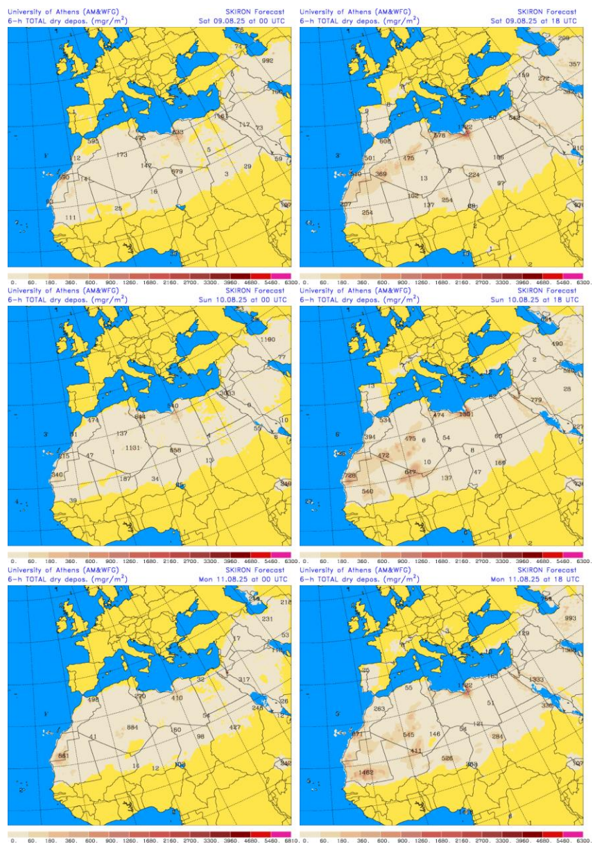
Depósito seco de polvo (mg/m 2 ) predicho por el modelo SKIRON para los días 9, 10 y 11 de agosto de 2025 a las 00 y 18 UTC © Universidad de Atenas.
