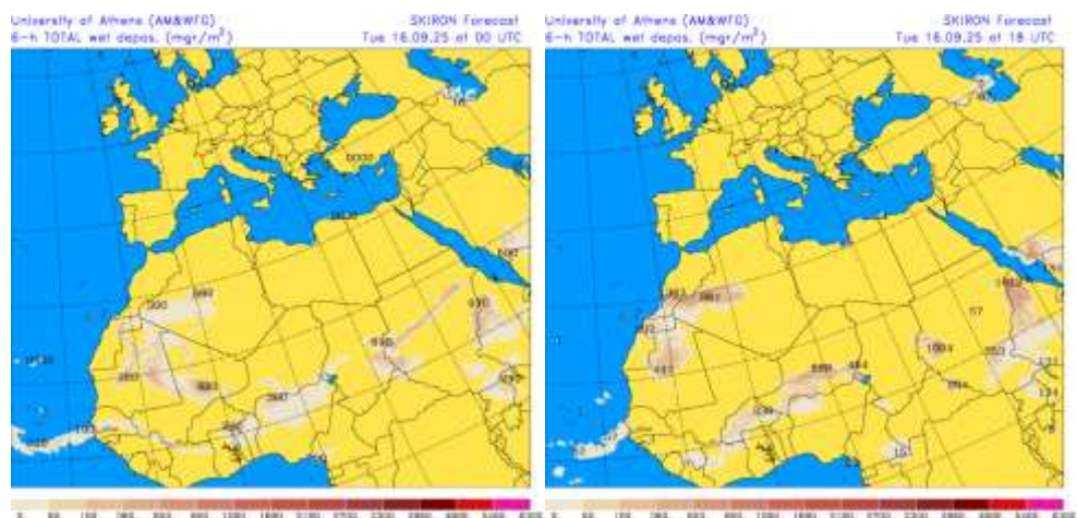
Depósito húmedo de polvo ( \text{mg}/\text{m}^2 ) predicho por el modelo SKIRON para el día 16 de septiembre de 2025 a las 00 y 18 UTC © Universidad de Atenas.
