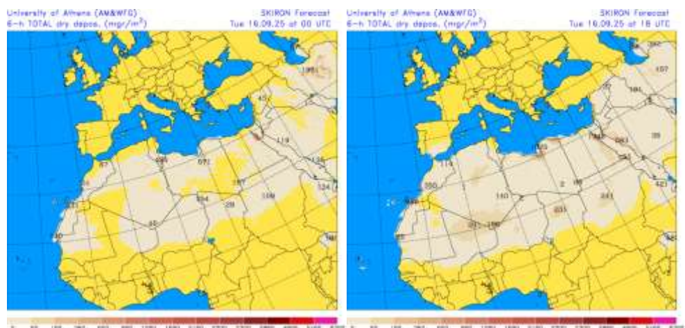
Depósito seco de polvo ( \text{mg}/\text{m}^2 ) predicho por el modelo SKIRON para el día 16 de septiembre de 2025 a las 00 y 18 UTC © Universidad de Atenas.
