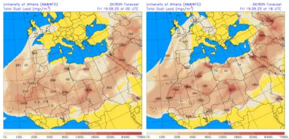
Carga total de polvo ( \text{mg}/\text{m}^2 ) predicha por el modelo SKIRON para el día 19 de septiembre de 2025 a las 00 y 18 UTC © Universidad de Atenas.
