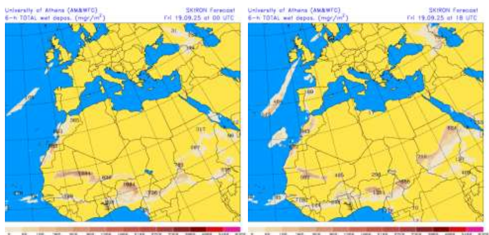
Depósito húmedo de polvo ( \text{mg}/\text{m}^2 ) predicho por el modelo SKIRON para el día 19 de septiembre de 2025 a las 00 y 18 UTC © Universidad de Atenas.
