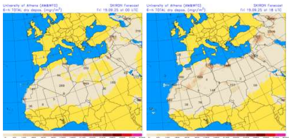
Depósito seco de polvo ( \text{mg}/\text{m}^2 ) predicho por el modelo SKIRON para el día 19 de septiembre de 2025 a las 00 y 18 UTC © Universidad de Atenas.
