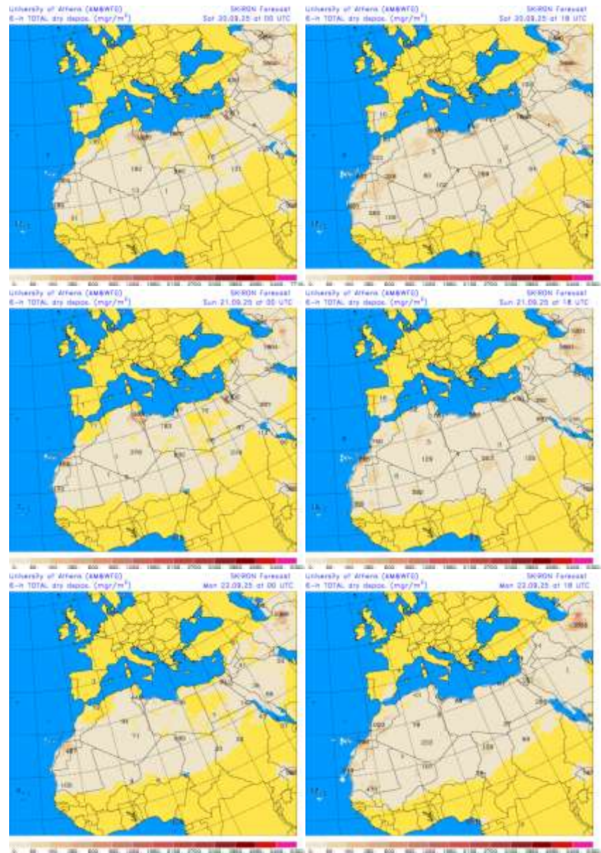
Depósito seco de polvo ( \text{mg}/\text{m}^2 ) predicho por el modelo SKIRON para los días 20, 21 y 22 de septiembre de 2025 a las 00 y 18 UTC © Universidad de Atenas.
