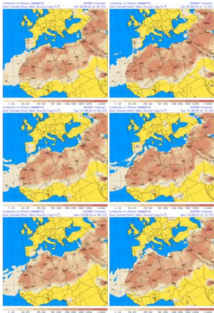
Concentración de polvo ( \mu\text{g}/\text{m}^3 ) predicha por el modelo SKIRON para los días 20, 21 y 22 de septiembre de 2025 a las 00 y 12 UTC © Universidad de Atenas.
