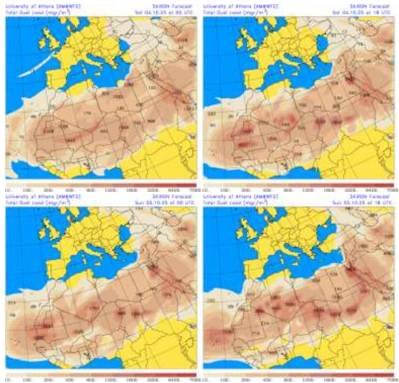
Carga total de polvo ( \text{mg}/\text{m}^2 ) predicha por el modelo SKIRON para los días 4 y 5 de octubre de 2025 a las 00 y 18 UTC © Universidad de Atenas.
