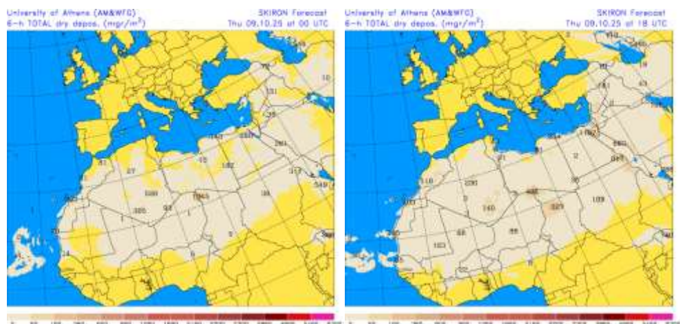
Depósito seco de polvo (mg/m²) predicho por el modelo SKIRON para el día 9 de octubre de 2025 a las 00 y 18 UTC © Universidad de Atenas.
