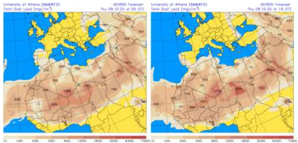
Carga total de polvo ( \text{mg}/\text{m}^2 ) predicha por el modelo SKIRON para el día 9 de octubre de 2025 a las 00 y 18 UTC © Universidad de Atenas.
