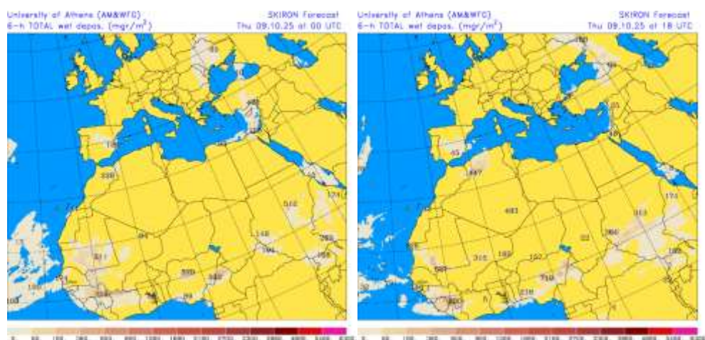
Depósito húmedo de polvo (mg/m²) predicho por el modelo SKIRON para el día 9 de octubre de 2025 a las 00 y 18 UTC © Universidad de Atenas.
