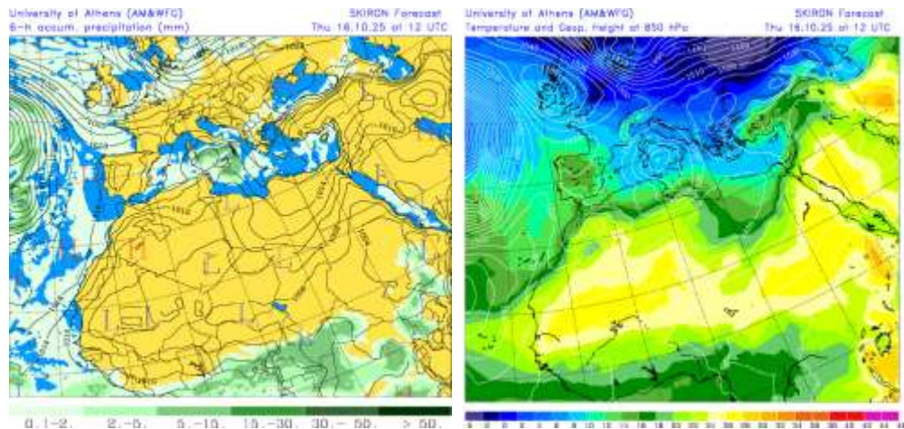
Precipitación acumulada (mm) y presión a nivel del mar (hPa) (izquierda) y campo de temperaturas (°C) y de altura geopotencial a 850 hPa (derecha) previsto por el modelo SKIRON para el día 16 de octubre de 2025 a las 12 UTC © Universidad de Atenas.
