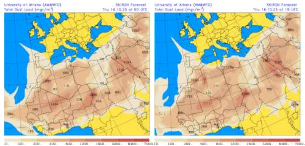
Carga total de polvo (mg/m 2 ) predicha por el modelo SKIRON para el día 16 de octubre de 2025 a las 00 y 18 UTC © Universidad de Atenas.
