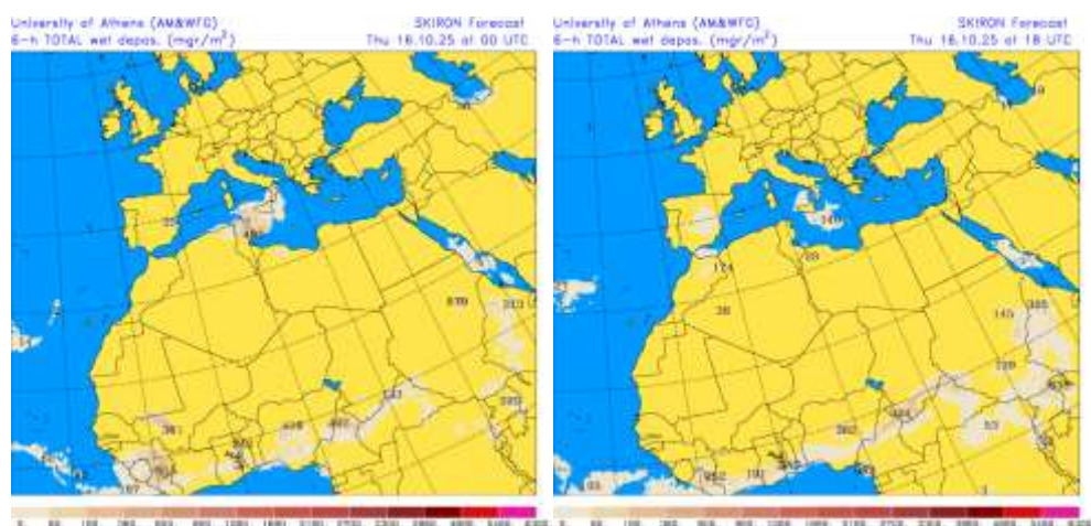
Depósito húmedo de polvo (mg/m 2 ) predicho por el modelo SKIRON para el día 16 de octubre de 2025 a las 00 y 18 UTC © Universidad de Atenas.
