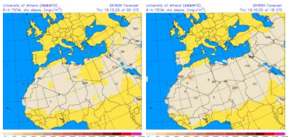
Depósito seco de polvo (mg/m 2 ) predicho por el modelo SKIRON para el día 16 de octubre de 2025 a las 00 y 18 UTC © Universidad de Atenas.
