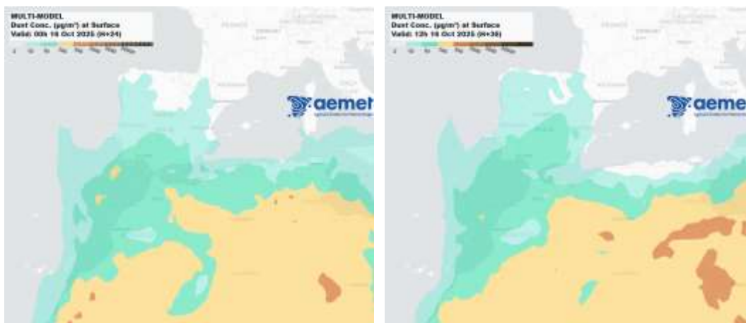
Resultado de la comparación de varios modelos de predicción de concentración de polvo ( \mu\text{g}/\text{m}^3 ) para el día 16 de octubre de 2025 a las 00h y 12h UTC. © Barcelona Dust Regional Center.
