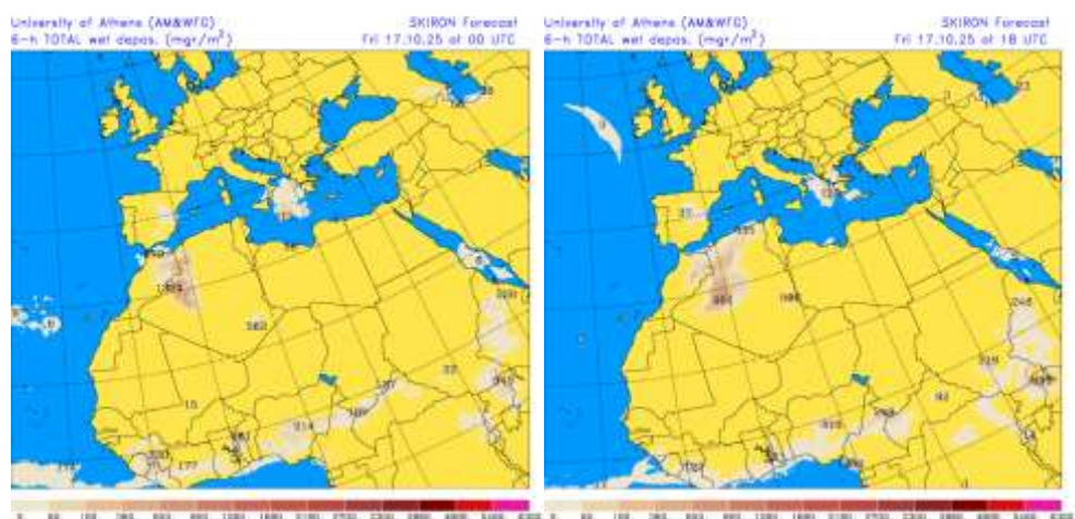
Depósito húmedo de polvo ( \text{mg}/\text{m}^2 ) predicho por el modelo SKIRON para el día 17 de octubre de 2025 a las 00 y 18 UTC © Universidad de Atenas.
