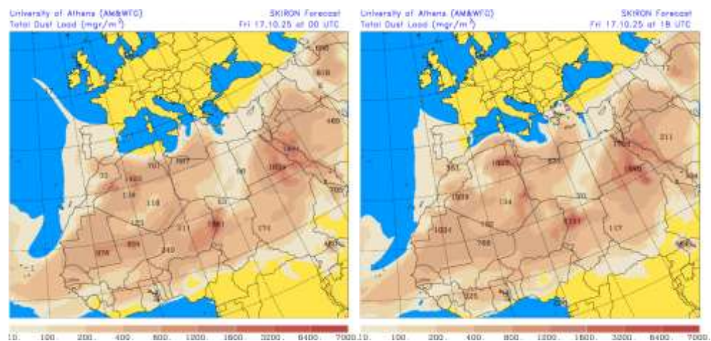
Carga total de polvo (mg/m 2 ) predicha por el modelo SKIRON para el día 17 de octubre de 2025 a las 00 y 18 UTC © Universidad de Atenas.
