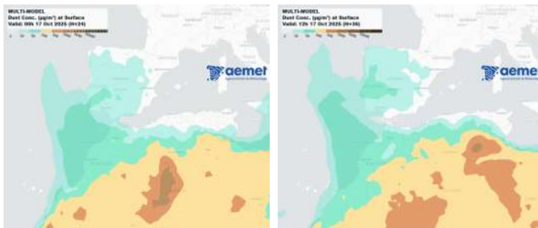
Resultado de la comparación de varios modelos de predicción de concentración de polvo ( \mu\text{g}/\text{m}^3 ) para el día 17 de octubre de 2025 a las 00h y 12h UTC. © Barcelona Dust Regional Center.
