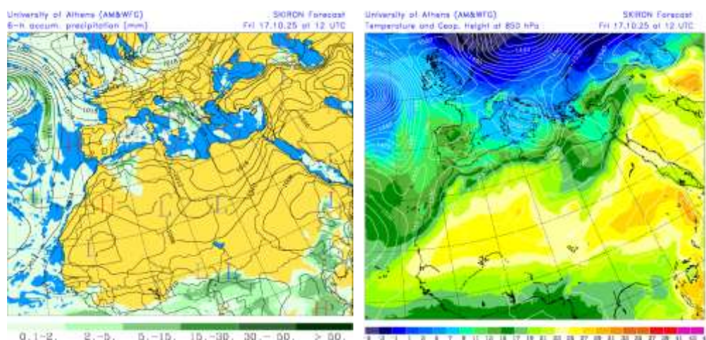
Precipitación acumulada (mm) y presión a nivel del mar (hPa) (izquierda) y campo de temperaturas (°C) y de altura geopotencial a 850 hPa (derecha) previsto por el modelo SKIRON para el día 17 de octubre de 2025 a las 12 UTC © Universidad de Atenas.
