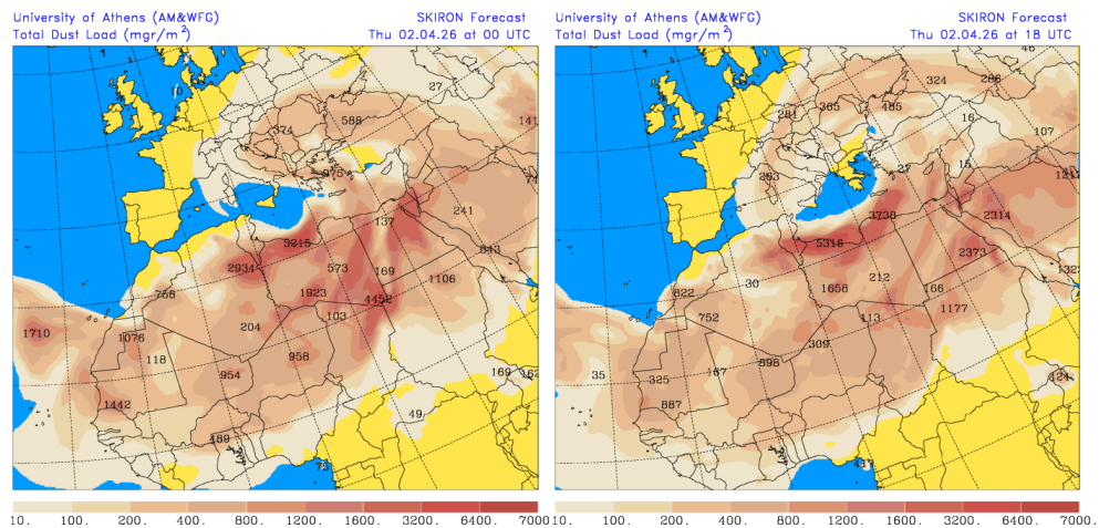
Carga total de polvo ( \text{mgr}/\text{m}^2 ) predicha por el modelo SKIRON para el día 2 de abril de 2026 a las 00 y 18 UTC © Universidad de Atenas.
