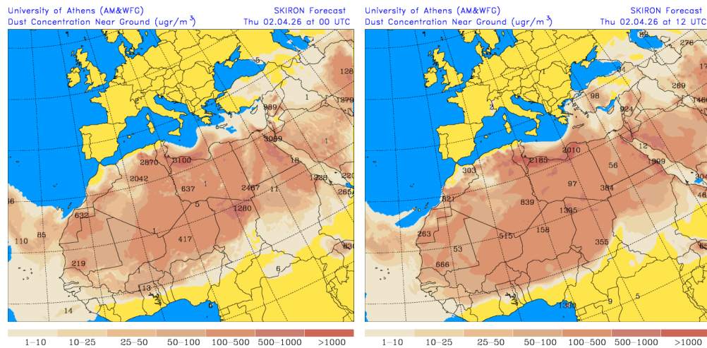
Concentración de polvo ( \mu\text{g}/\text{m}^3 ) predicha por el modelo SKIRON para el día 2 de abril de 2026 a las 00 y 12 UTC © Universidad de Atenas.
