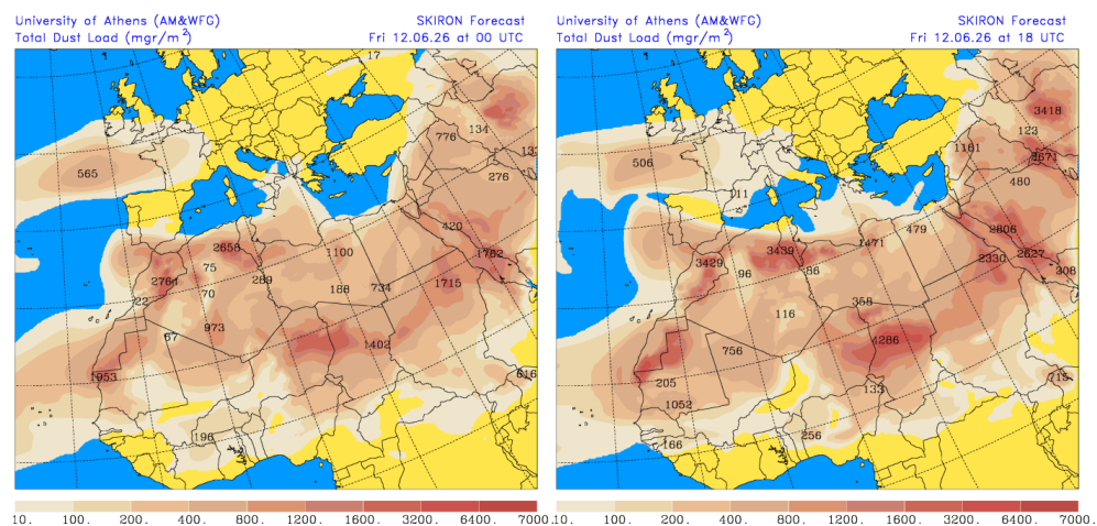
Carga total de polvo (mg/m 2 ) predicha por el modelo SKIRON para el día 12 de junio de 2026 a las 00 y 18 UTC © Universidad de Atenas.
