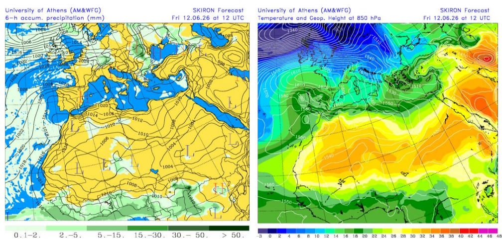
Precipitación acumulada (mm) y presión a nivel del mar (hPa) (izquierda) y campo de temperaturas (°C) y de altura geopotencial a 850 hPa (derecha) previsto por el modelo SKIRON para el día 12 de junio de 2026 a las 12 UTC © Universidad de Atenas.
