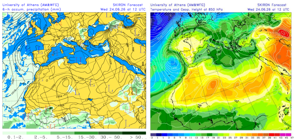
Precipitación acumulada (mm) y presión a nivel del mar (hPa) (izquierda) y campo de temperaturas (°C) y de altura geopotencial a 850 hPa (derecha) previsto por el modelo SKIRON para el día 24 de junio de 2026 a las 12 UTC © Universidad de Atenas.
