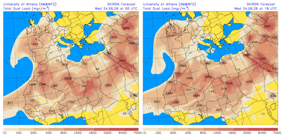
Carga total de polvo (mg/m 2 ) predicha por el modelo SKIRON para el día 24 de junio de 2026 a las 00 y 18 UTC © Universidad de Atenas.
