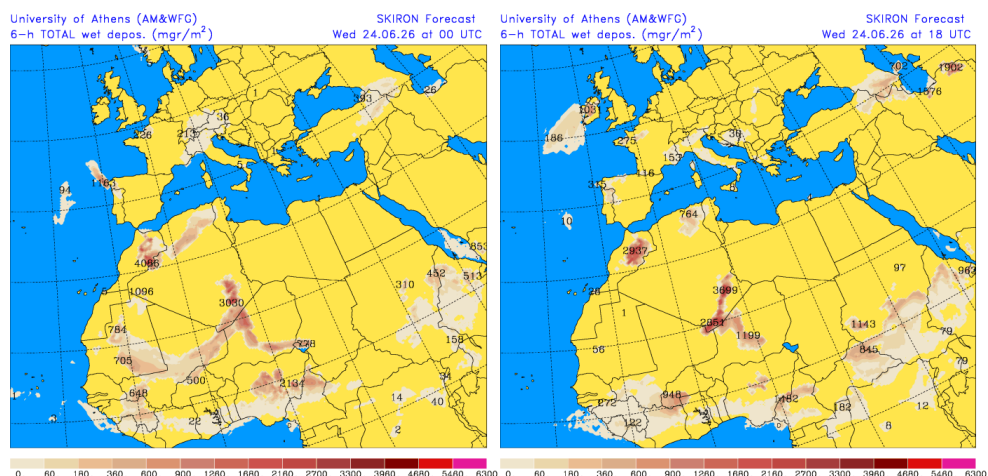
Depósito húmedo de polvo (mg/m 2 ) predicho por el modelo SKIRON para el día 24 de junio de 2026 a las 00 y 18 UTC © Universidad de Atenas.
