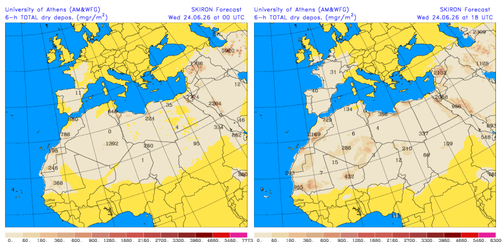
Depósito seco de polvo (mg/m 2 ) predicho por el modelo SKIRON para el día 24 de junio de 2026 a las 00 y 18 UTC © Universidad de Atenas.
