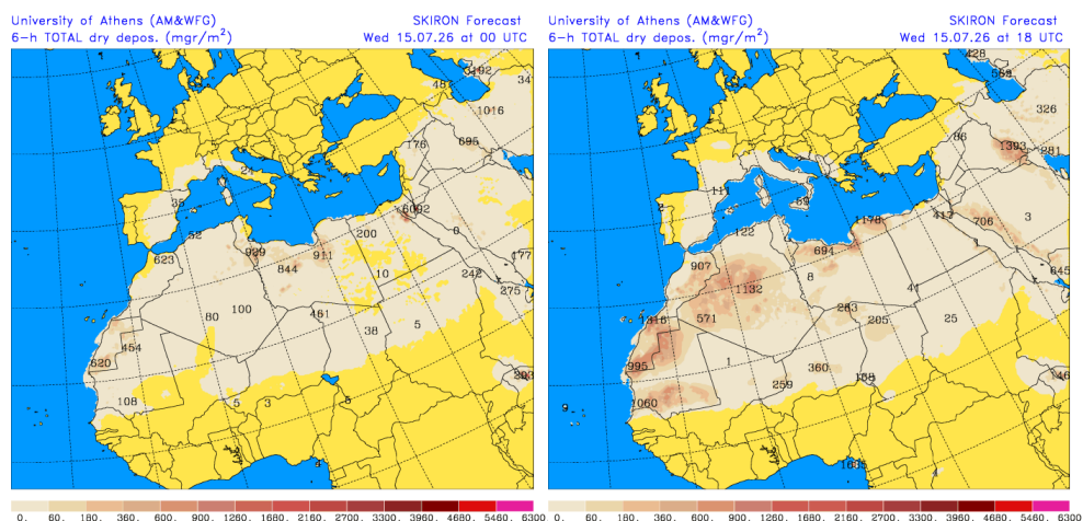
Depósito seco de polvo (mg/m 2 ) predicho por el modelo SKIRON para el día 15 de julio de 2026 a las 00 y 18 UTC © Universidad de Atenas.
