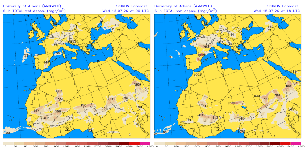
Depósito húmedo de polvo (mg/m 2 ) predicho por el modelo SKIRON para el día 15 de julio de 2026 a las 00 y 18 UTC © Universidad de Atenas.
