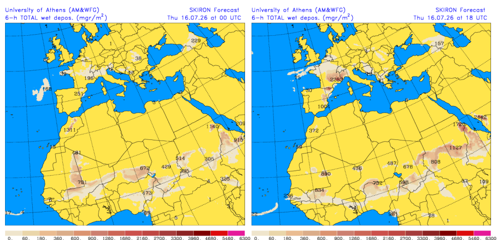
Depósito húmedo de polvo ( \text{mg}/\text{m}^2 ) predicho por el modelo SKIRON para el día 16 de julio de 2026 a las 00 y 18 UTC © Universidad de Atenas.
