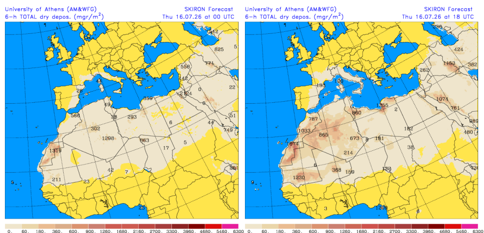
Depósito seco de polvo ( \text{mg}/\text{m}^2 ) predicho por el modelo SKIRON para el día 16 de julio de 2026 a las 00 y 18 UTC © Universidad de Atenas.
