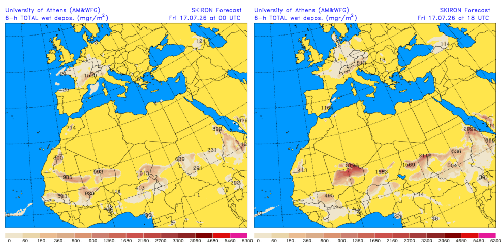
Depósito húmedo de polvo (mg/m 2 ) predicho por el modelo SKIRON para el día 17 de julio de 2026 a las 00 y 18 UTC © Universidad de Atenas.
