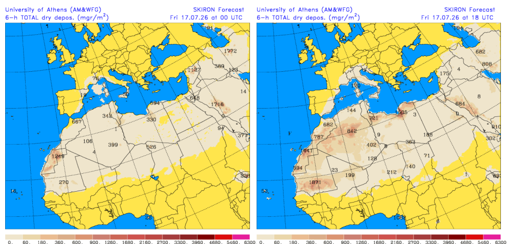
Depósito seco de polvo (mg/m 2 ) predicho por el modelo SKIRON para el día 17 de julio de 2026 a las 00 y 18 UTC © Universidad de Atenas.
