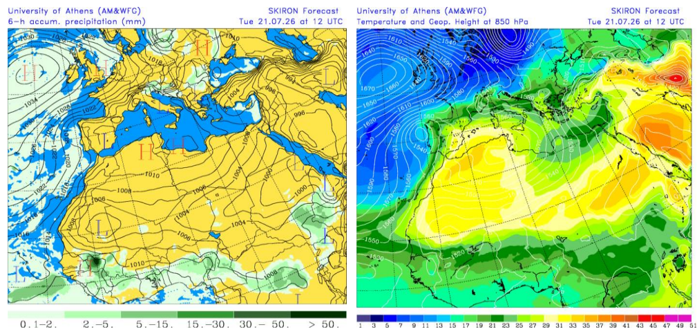
Precipitación acumulada (mm) y presión a nivel del mar (hPa) (izquierda) y campo de temperaturas (°C) y de altura geopotencial a 850 hPa (derecha) previsto por el modelo SKIRON para el día 21 de julio de 2026 a las 12 UTC © Universidad de Atenas.
