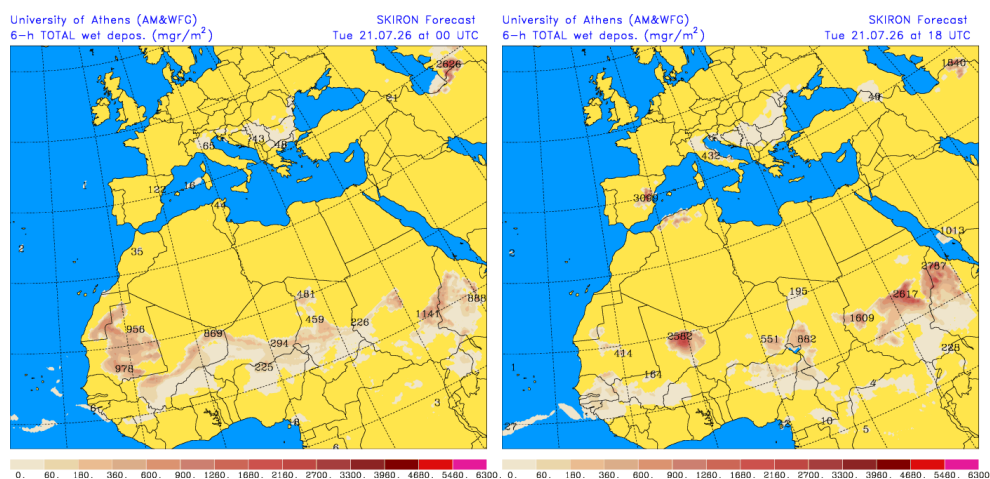
Depósito húmedo de polvo ( \text{mg}/\text{m}^2 ) predicho por el modelo SKIRON para el día 21 de julio de 2026 a las 00 y 18 UTC © Universidad de Atenas.
