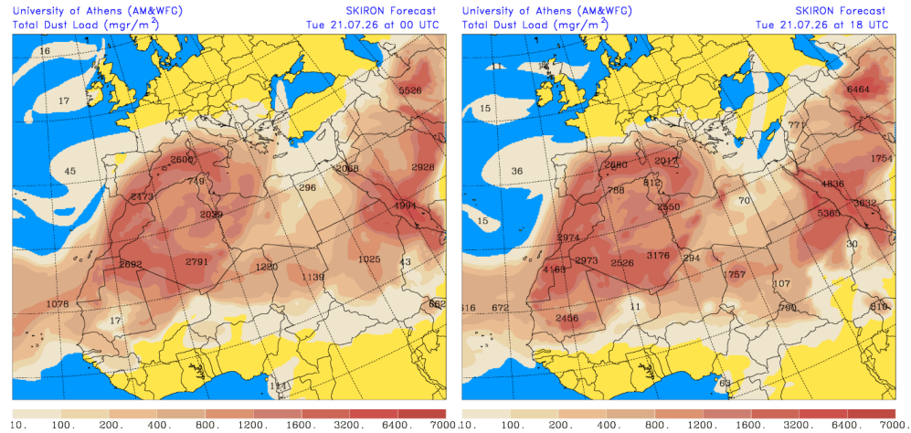
Carga total de polvo (mg/m 2 ) predicha por el modelo SKIRON para el día 21 de julio de 2026 a las 00 y 18 UTC © Universidad de Atenas.
