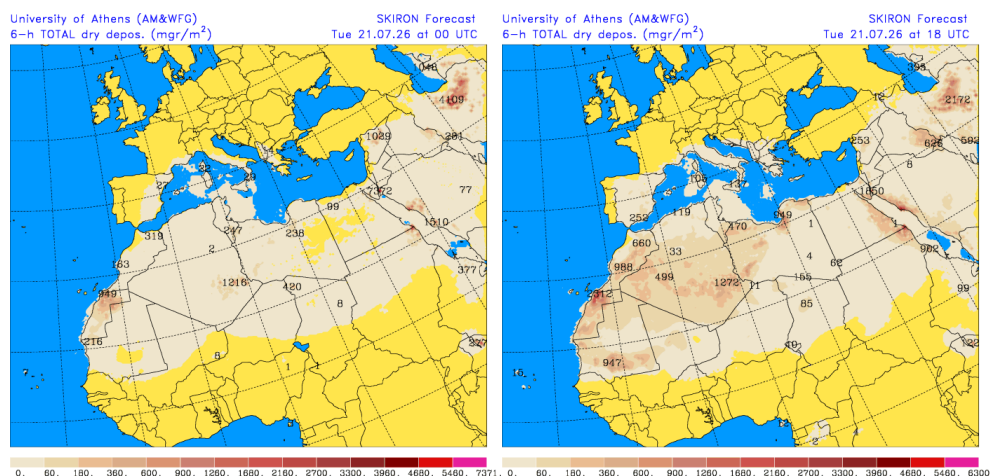
Depósito seco de polvo ( \text{mg}/\text{m}^2 ) predicho por el modelo SKIRON para el día 21 de julio de 2026 a las 00 y 18 UTC © Universidad de Atenas.
