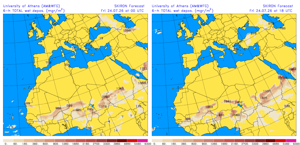
Depósito húmedo de polvo (mg/m 2 ) predicho por el modelo SKIRON para el día 24 de julio de 2026 a las 00 y 18 UTC © Universidad de Atenas.
