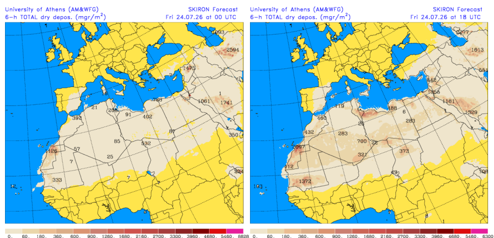
Depósito seco de polvo (mg/m 2 ) predicho por el modelo SKIRON para el día 24 de julio de 2026 a las 00 y 18 UTC © Universidad de Atenas.
