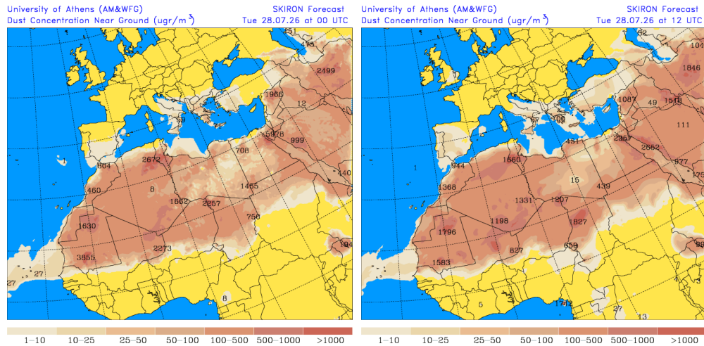
Concentración de polvo ( \mu\text{g}/\text{m}^3 ) predicha por el modelo SKIRON para el día 28 de julio de 2026 a las 00 y 12 UTC © Universidad de Atenas.
