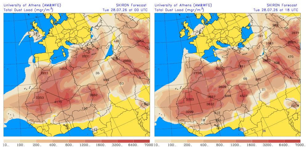
Carga total de polvo ( \text{mg}/\text{m}^2 ) predicha por el modelo SKIRON para el día 28 de julio de 2026 a las 00 y 18 UTC © Universidad de Atenas.
