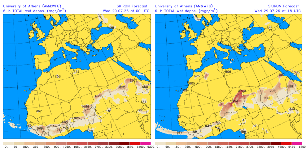
Depósito húmedo de polvo ( \text{mg}/\text{m}^2 ) predicho por el modelo SKIRON para el día 29 de julio de 2026 a las 00 y 18 UTC © Universidad de Atenas.
