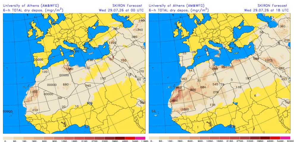
Depósito seco de polvo ( \text{mg}/\text{m}^2 ) predicho por el modelo SKIRON para el día 29 de julio de 2026 a las 00 y 18 UTC © Universidad de Atenas.
