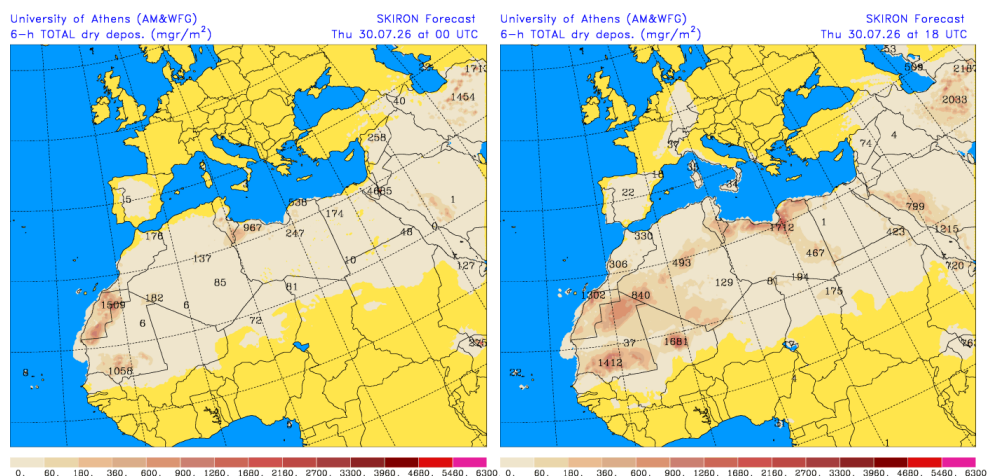
Depósito seco de polvo ( \text{mg}/\text{m}^2 ) predicho por el modelo SKIRON para el día 30 de julio de 2026 a las 00 y 18 UTC © Universidad de Atenas.
