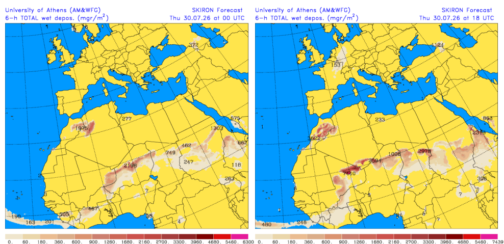
Depósito húmedo de polvo ( \text{mg}/\text{m}^2 ) predicho por el modelo SKIRON para el día 30 de julio de 2026 a las 00 y 18 UTC © Universidad de Atenas.
