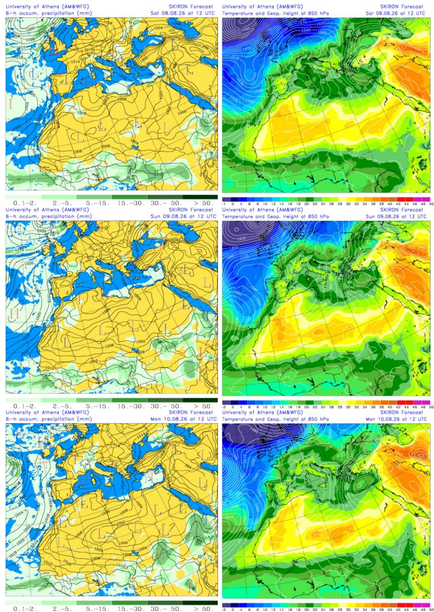
Precipitación acumulada (mm) y presión a nivel del mar (hPa) (izquierda) y campo de temperaturas (°C) y de altura geopotencial a 850 hPa (derecha) previsto por el modelo SKIRON para los días 8, 9 y 10 de agosto de 2026 a las 12 UTC © Universidad de Atenas.
