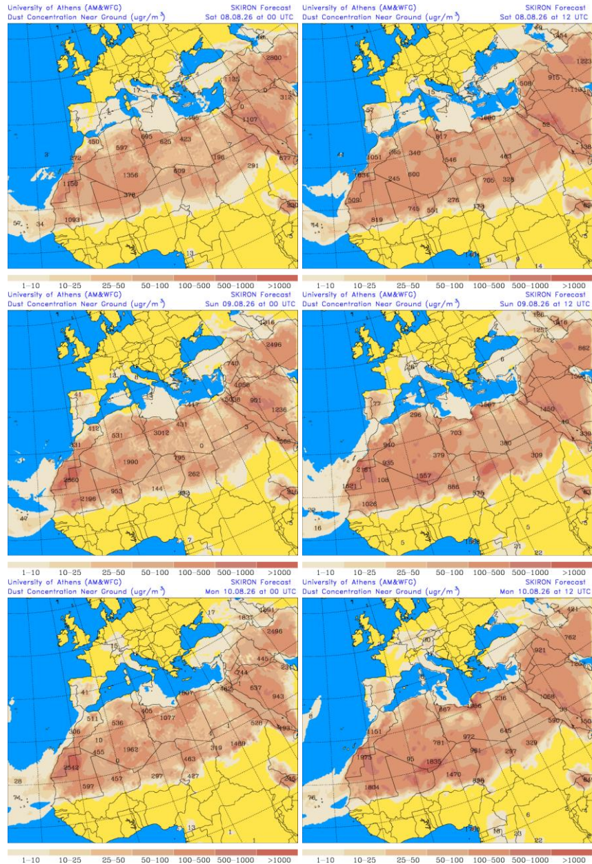
Concentración de polvo ( \mu\text{g}/\text{m}^3 ) predicha por el modelo SKIRON para los días 8, 9 y 10 de agosto de 2026 a las 00 y 12 UTC © Universidad de Atenas.
