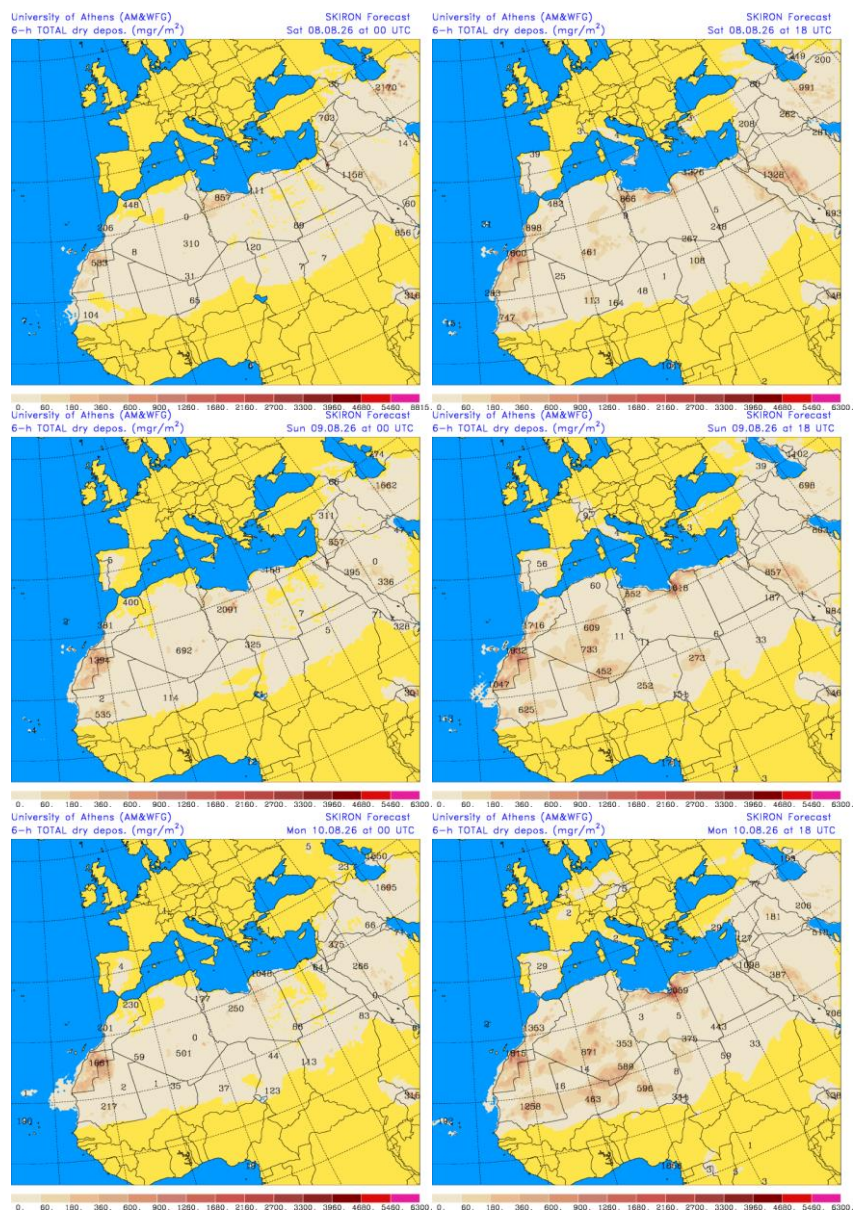
Depósito seco de polvo (mg/m 2 ) predicho por el modelo SKIRON para los días 8, 9 y 10 de agosto de 2026 a las 00 y 18 UTC © Universidad de Atenas.
