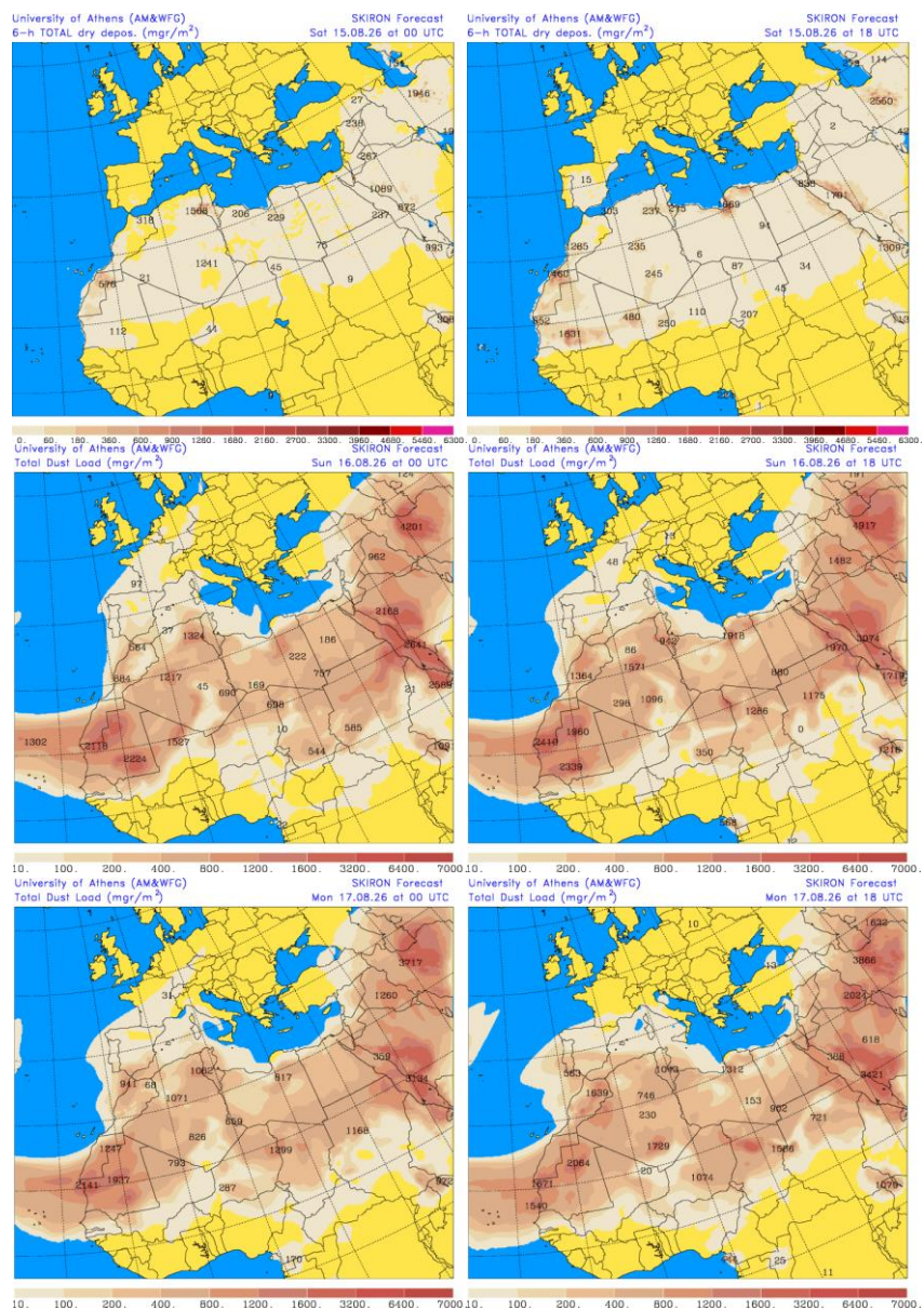
Depósito seco de polvo (mg/m 2 ) predicho por el modelo SKIRON para los días 15, 16 y 17 de agosto de 2026 a las 00 y 18 UTC © Universidad de Atenas.
