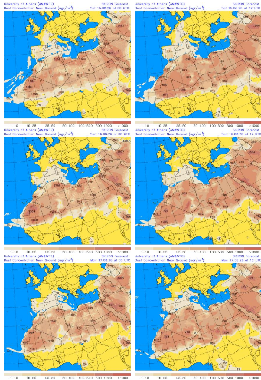
Concentración de polvo ( \mu\text{g}/\text{m}^3 ) predicha por el modelo SKIRON para los días 15, 16 y 17 de agosto de 2026 a las 00 y 12 UTC © Universidad de Atenas.
