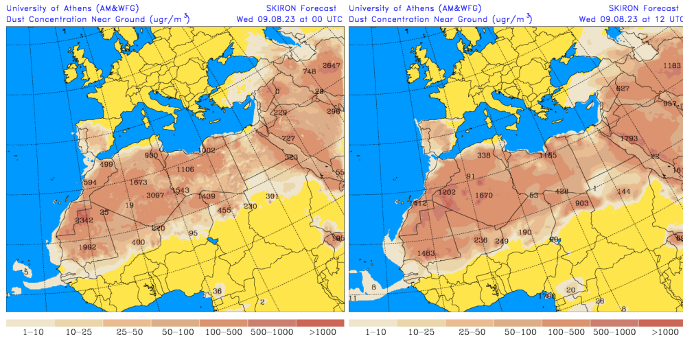
Concentración de polvo ( \mu\text{g}/\text{m}^3 ) predicha por el modelo SKIRON para el día 09 de agosto de 2023 a las 00 y 12 UTC © Universidad de Atenas.
