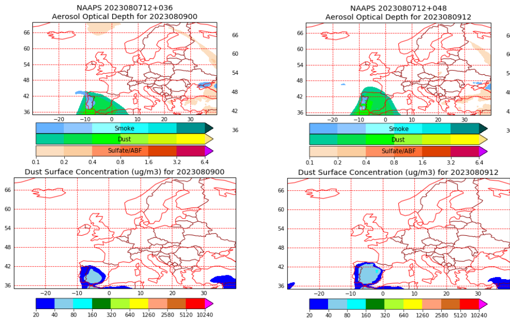
Espesor óptico de aerosoles a 550 nm (arriba) y concentración de polvo a nivel de superficie (abajo) previstos por el modelo NAAPS para el día 09 de agosto de 2023 a las 00 h UTC y a las 12 h UTC. ©Naval Research Laboratory (NRL), Monterey, CA.
