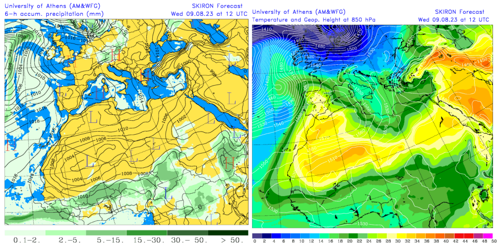
Precipitación acumulada (mm) y presión a nivel del mar (hPa) (izquierda) y campo de temperaturas (°C) y de altura geopotencial a 850 hPa (derecha) previsto por el modelo SKIRON para el día 09 de agosto de 2023 a las 12 UTC © Universidad de Atenas.
