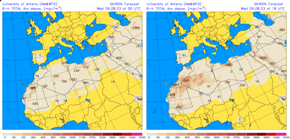
Depósito seco de polvo ( \text{mg}/\text{m}^2 ) predicho por el modelo SKIRON para el día 09 de agosto de 2023 a las 00 y 18 UTC © Universidad de Atenas.
