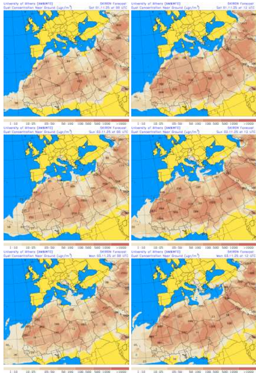
Concentración de polvo ( \mu\text{g}/\text{m}^3 ) predicha por el modelo SKIRON para los días 1, 2 y 3 de noviembre de 2025 a las 00 y 12 UTC © Universidad de Atenas.
