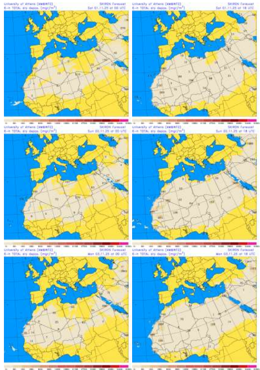
Depósito seco de polvo ( \text{mg}/\text{m}^2 ) predicho por el modelo SKIRON para los días 1, 2 y 3 de noviembre de 2025 a las 00 y 18 UTC © Universidad de Atenas.
