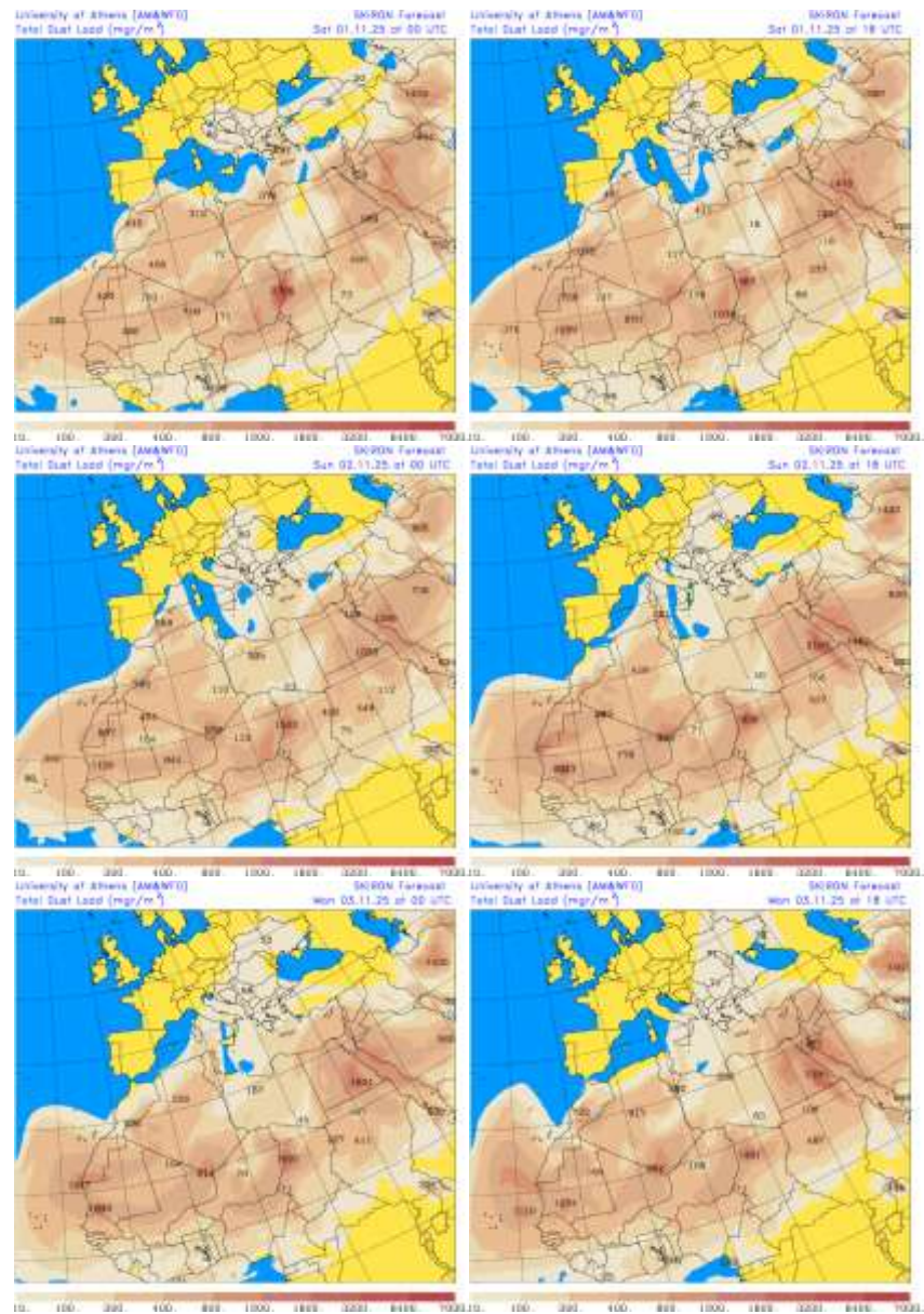
Carga total de polvo (mg/m²) predicha por el modelo SKIRON para los días 1, 2 y 3 de noviembre de 2025 a las 00 y 18 UTC © Universidad de Atenas.
