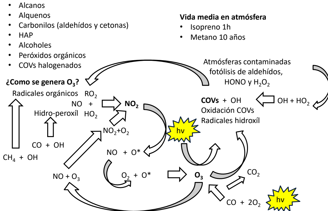
Figura 1. Esquema mostrando el ciclo del O 3 y los sub-productos generados.
