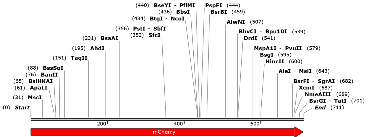
mCherry 711 bp
