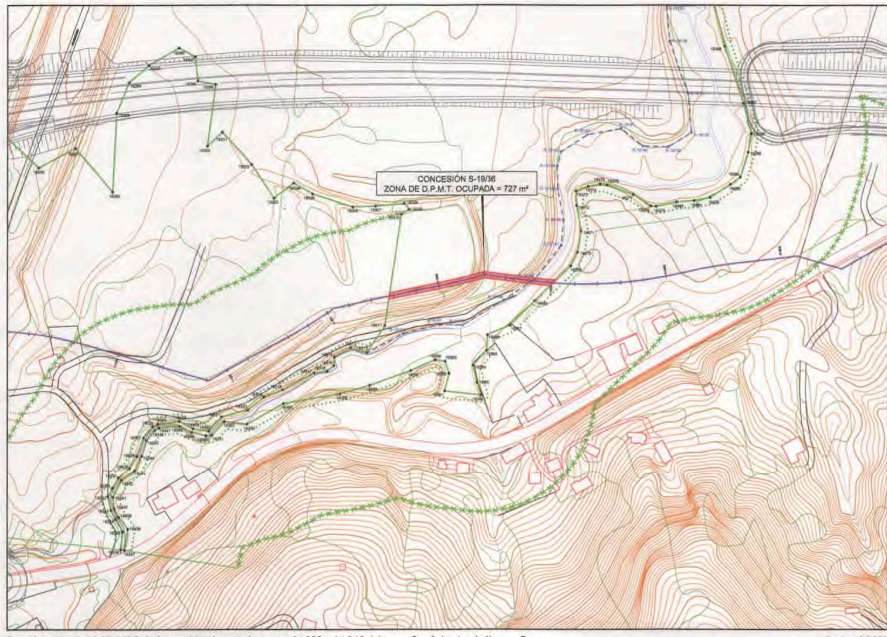
Zona de ocupación del D.P.M.T. de la canalización entre los puntos 1+098 y 1+245 del tramo San Salvador de Heras - Camargo. Escala = 1:2,000
