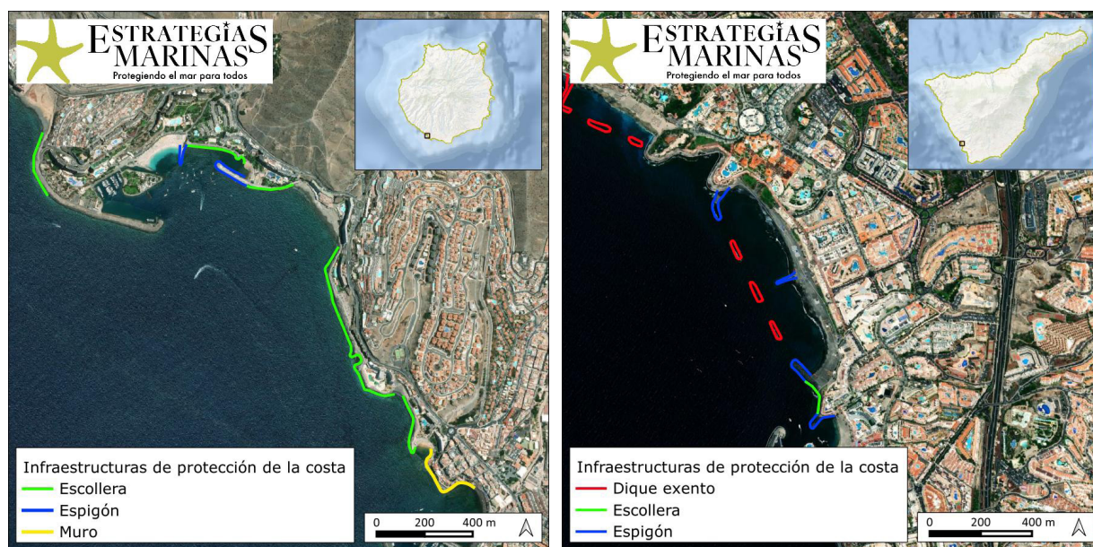
Figura 5. Detalle de los elementos de protección de la costa presentes en Mogán, Gran Canaria (izquierda) y Adeje, Tenerife (derecha). (Fuente: CEDEX).
