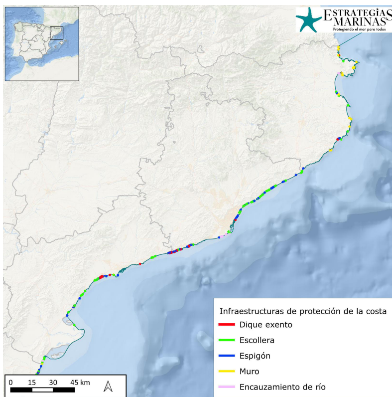
Figura 8. Localización de las infraestructuras de protección de la costa existentes en Cataluña. (Fuente: CEDEX).
