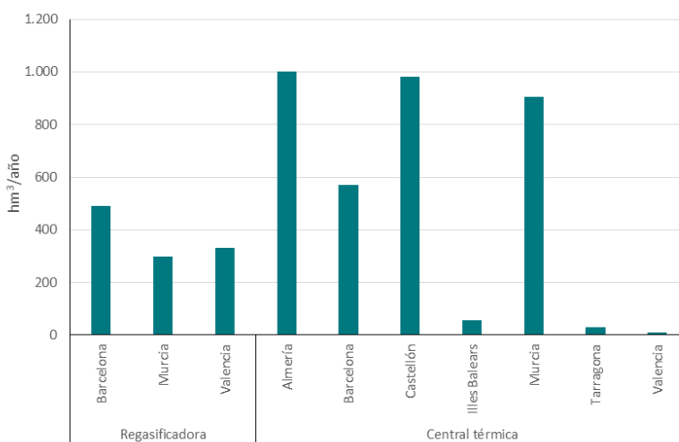
Figura 39. Caudales de captación teóricos de agua de mar de las centrales térmicas y regasificadoras en el periodo 2016-2021 en la demarcación marina levantino-balear. (Fuente: PRTR)
