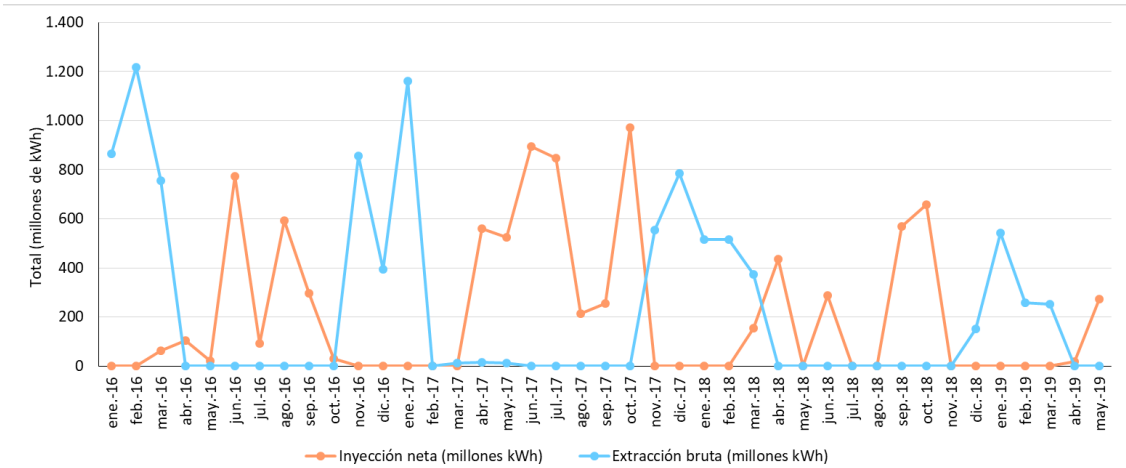
Figura 25. Inyección y extracción del almacenamiento Gaviota durante los años 2016 y 2019. (Fuente: Figura elaborada por el CEDEX a partir de datos de Enagas)
